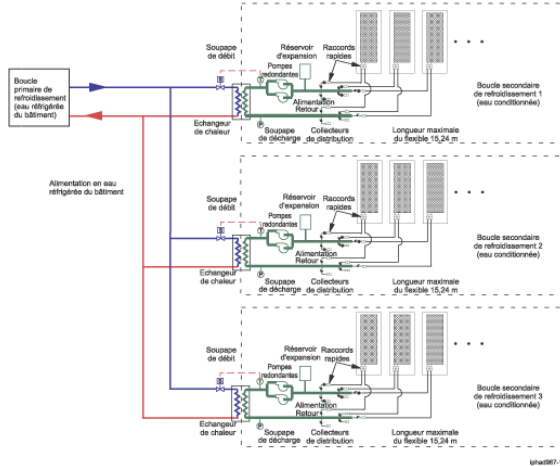
Figure 3. Boucles primaires et secondaires de refroidissement
