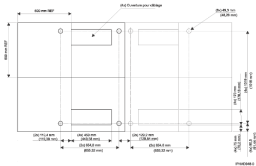
Figure 2. Positionnement des boulons à oeil pour dalles de plancher de 600 mm
