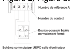
Figure 2. Figure de connecteur AMP
