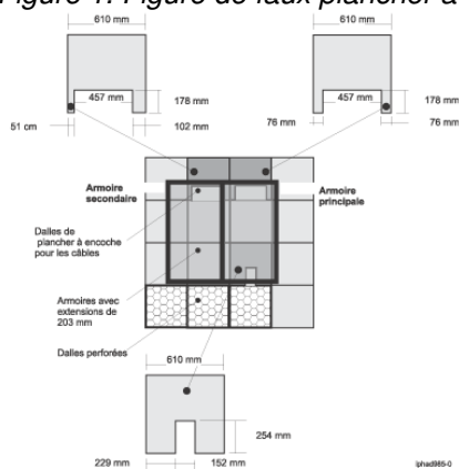
Figure 1. Figure de faux plancher avec dalles de 610 mm
