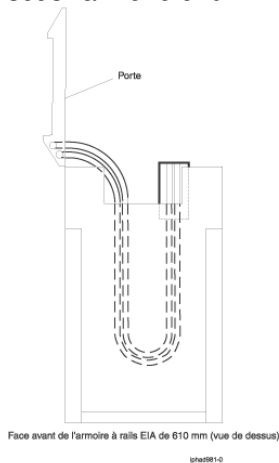
Figure 8. Exemple 2 - Gestion des tuyaux dans des environnements avec ou sans faux plancher - Boucle sous l'armoire 610 mm (24 pouces) à rails EIA (porte ouverte)
