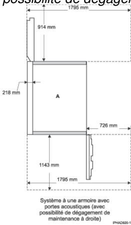
Figure 5. Dégagements de maintenance pour un système à une armoire muni de portes acoustiques (avec possibilité de dégagement de maintenance à droite)
