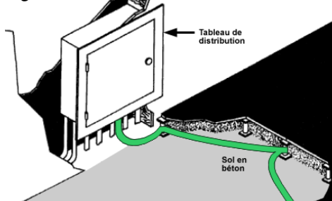
Figure 3. Mise à la terre transitoire à l'aide de la structure supportant le faux plancher
