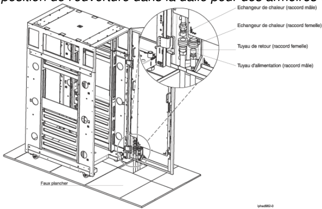
Figure 2. Exemple 1 - Gestion des tuyaux dans un environnement avec faux plancher - Dimensions et position de l'ouverture dans la dalle pour des armoires 610 mm (24 pouces) à rails EIA
