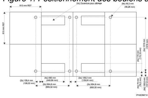
Figure 1. Positionnement des boulons à oeil pour dalles de plancher de 610 mm
