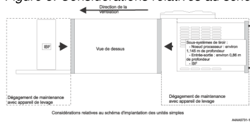
Figure 5. Considérations relatives au schéma d'implantation des unités simples
