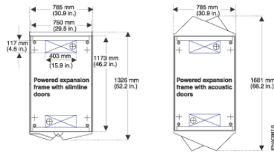
Figure 1. Vue de dessus pour systèmes à une armoire avec portes extra-plates et acoustiques
