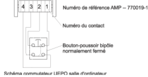
Figure 2. Figure de connecteur AMP
