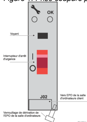
Figure 1. Prise coupure par arrêt d'urgence
