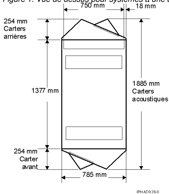
Figure 1. Vue de dessus pour systèmes à une armoire avec portes acoustiques
