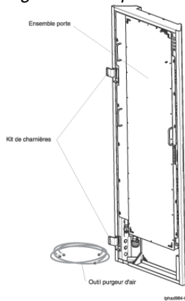
Figure 2. Composants du kit d'options d'échangeur de chaleur pour armoires 610 mm (24 pouces) à rails EIA
