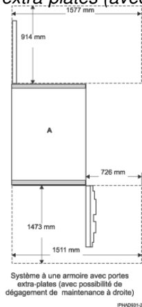
Figure 2. Dégagements de maintenance pour les systèmes 185/75 à une armoire munis de portes extra-plates (avec possibilité de dégagement de maintenance à droite)
