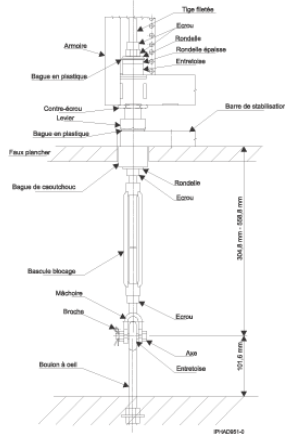
Figure 6. Matériel d'ancrage d'assemblage de lanterne de tendeur pour un faux plancher de 304,8 mm à 558,8 mm (44P3000)
