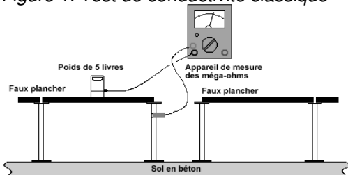
Figure 1. Test de conductivité classique
