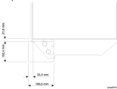
Figure 3. Exemple 1 - Gestion des tuyaux dans un environnement avec faux plancher - Définition et emplacement de l'ouverture dans la dalle pour des armoires 483 mm (19 pouces) à rails EIA
