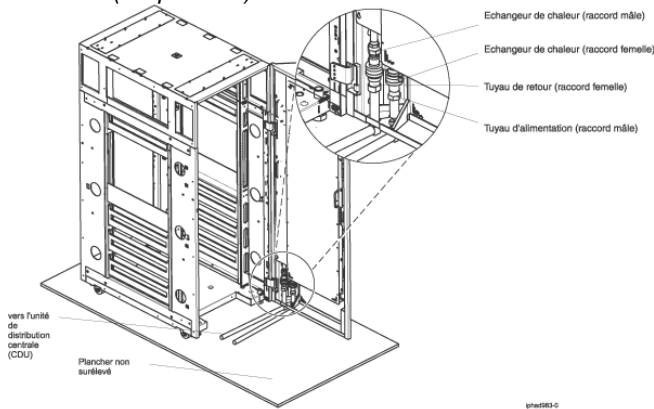
Figure 2. Spécifications relatives à la tuyauterie dans un environnement sans faux plancher pour une armoire 610 mm (24 pouces) à rails EIA
