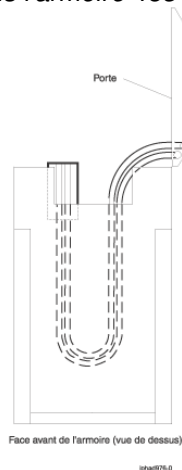
Figure 7. Exemple 2 - Gestion des tuyaux dans des environnements avec ou sans faux plancher - Boucle sous l'armoire 483 mm (19 pouces) à rails EIA (porte ouverte)
