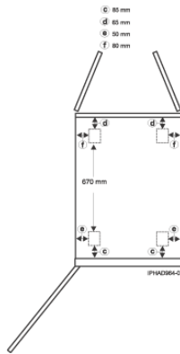
Emplacements des roulettes des modèles 05/55 et 14S/25
