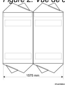
Figure 2. Vue de dessus pour systèmes à deux armoires avec portes acoustiques
