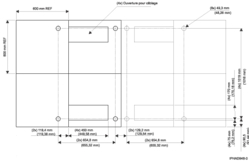
Figure 2. Positionnement des boulons à œil pour dalles de plancher de 600 mm
