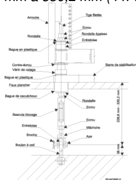
Figure 4. Matériel d'ancrage d'assemblage de lanterne de tendeur pour un faux plancher de 228,6 mm à 330,2 mm (44P2999)
