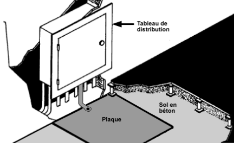
Figure 2. Prise de mise à la terre transitoire
