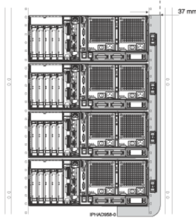
Figure 3. Schéma d'insertion de l'assemblage flexible du modèle ESCALA PL 850R/PL 1650R/R+ (vue arrière)
