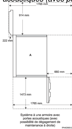
Figure 4. Dégagements de maintenance pour les systèmes 185/75 à une armoire munis de portes acoustiques (avec possibilité de dégagement de maintenance à droite)
