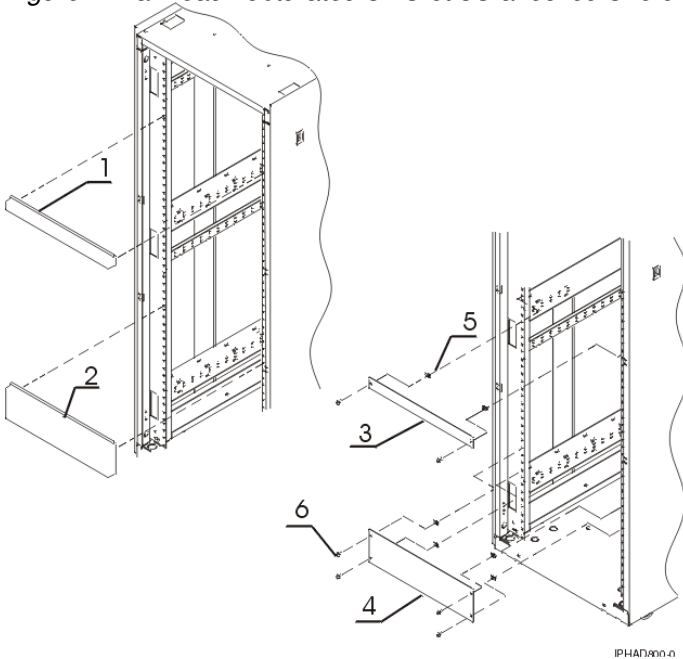
Figure 1. Panneaux obturateurs 1U et 3U avec leurs références
