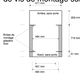
Figure 1. Vue de dessus des spécifications de dimension d'une armoire Vue de dessus des spécifications de dimension d'une armoire
