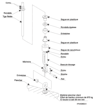
Figure 6. Matériel d'ancrage d'assemblage de lanterne de tendeur pour un faux plancher de 304,8 mm à 558,8 mm (44P3000)
