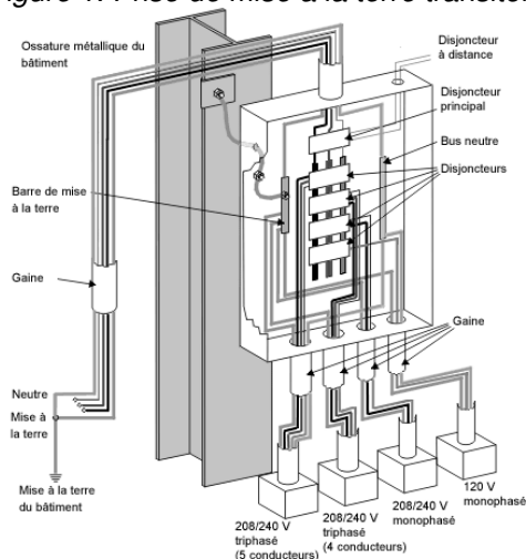
Figure 1. Prise de mise à la terre transitoire
