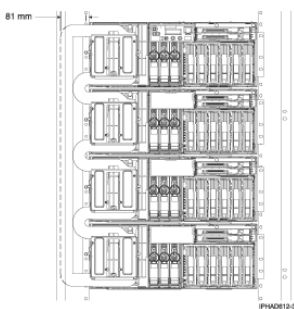
Figure 2. Schéma d'insertion de l'assemblage flexible du modèle ESCALA PL 850R/PL 1650R/R+ (vue avant)
