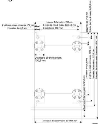
Figure 3. Pied de nivellement et dimensions de l'armoire
