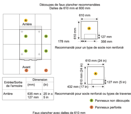
Figure 1. Faux plancher avec dalles de 610 mm
