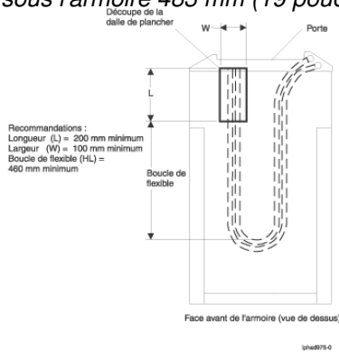
Figure 5. Exemple 2 - Gestion des tuyaux dans des environnements avec ou sans faux plancher - Boucle sous l'armoire 483 mm (19 pouces) à rails EIA (porte fermée)
