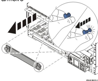
Figure 2. Panneau obturateur de la carte d'activation RAID dans une unité centrale montée en armoire
