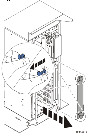
Figure 1. Panneau obturateur de la carte d'activation RAID dans une unité centrale autonome
