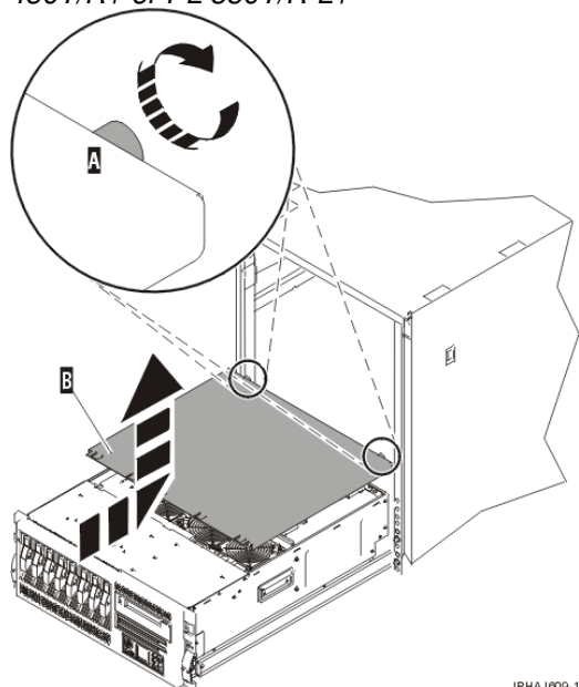
Figure 1. Retrait du capot d'accès du modèle monté en armoire ESCALA PL 250T/R, ESCALA PL 450T/R, PL 450T/R+ or PL 850T/R-L+
