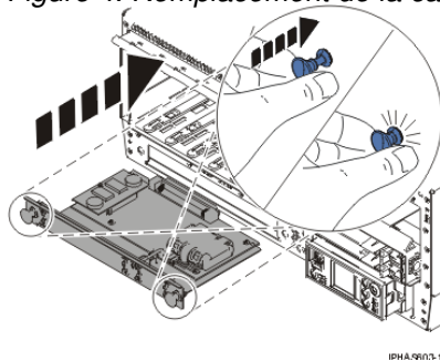
Figure 4. Remplacement de la carte d'activation RAID dans une unité centrale montée en armoire
