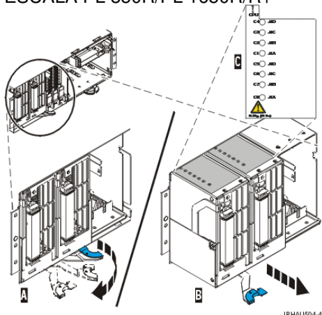
Figure 1. Retrait du fond de panier système de l'unité centrale du modèle ESCALA PL 1650R-L+ ou ESCALA PL 850R/PL 1650R/R+
