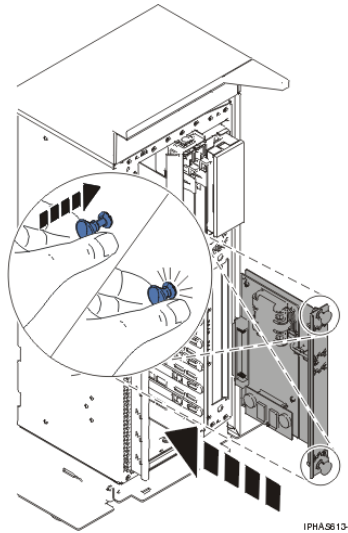
Figure 4. Remplacement de la carte d'activation RAID dans une unité centrale montée en armoire
