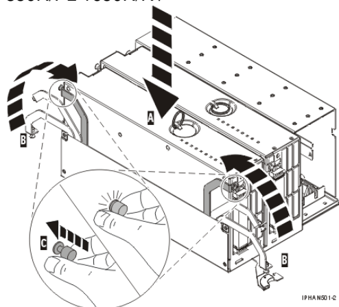
Figure 1. Remplacement du fond de panier du modèle ESCALA PL 1650R-L+ ou ESCALA PL 850R/PL 1650R/R+
