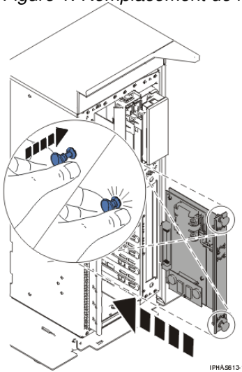
Figure 1. Remplacement de la carte d'activation RAID dans une unité centrale autonome
