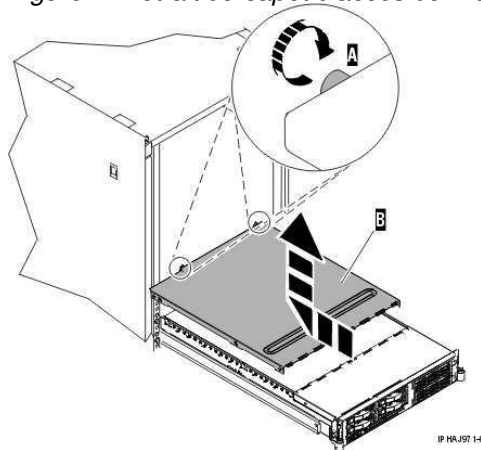
Figure 2. Retrait du capot d'accès du modèle ESCALA PL 250R-L, PL 250R-L+ or PL 450R-VL+ ou 7/10
