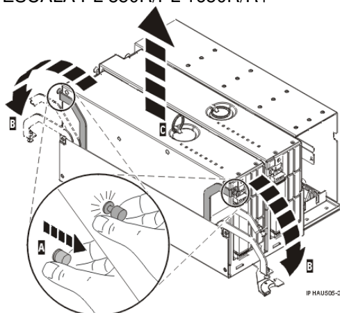
Figure 2. Retrait du bloc processeur du fond de panier système du modèle ESCALA PL 1650R-L+ ou ESCALA PL 850R/PL 1650R/R+
