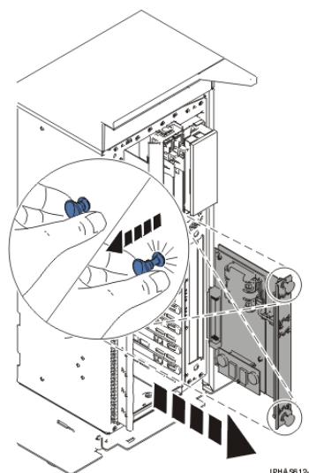
Figure 2. Retrait de la carte d'activation RAID dans une unité centrale montée en armoire
