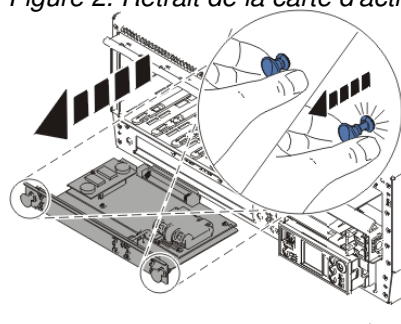
Figure 2. Retrait de la carte d'activation RAID dans une unité centrale montée en armoire
