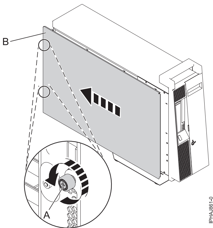
Figure 19. Retrait du capot d'accès d'un modèle autonome
