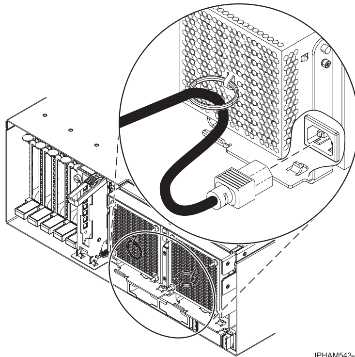
Figure 5. Passage du câble dans l'anneau de l'alimentation électrique
