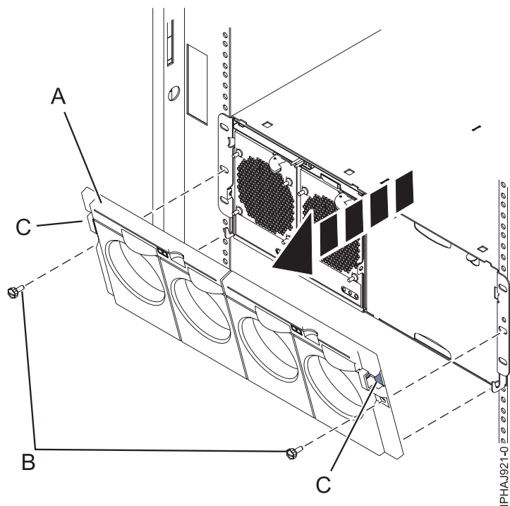
Figure 14. Panneau avant sur un modèle 14G/30
