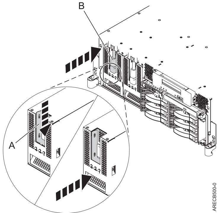
Figure 8. Remplacement d'une alimentation électrique
