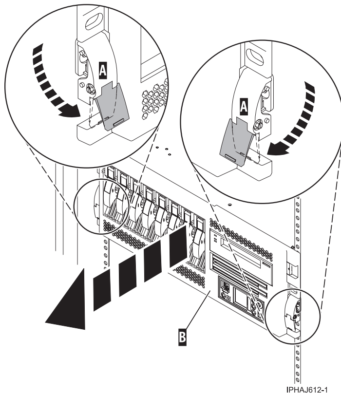
Figure 28. Libération des loquets de sécurité
