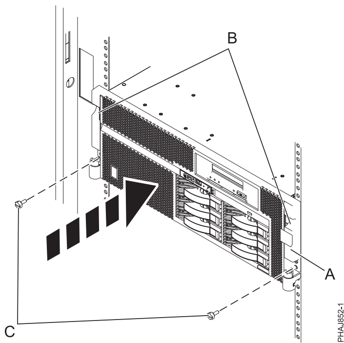
Figure 33. Remplacement des vis moletées
