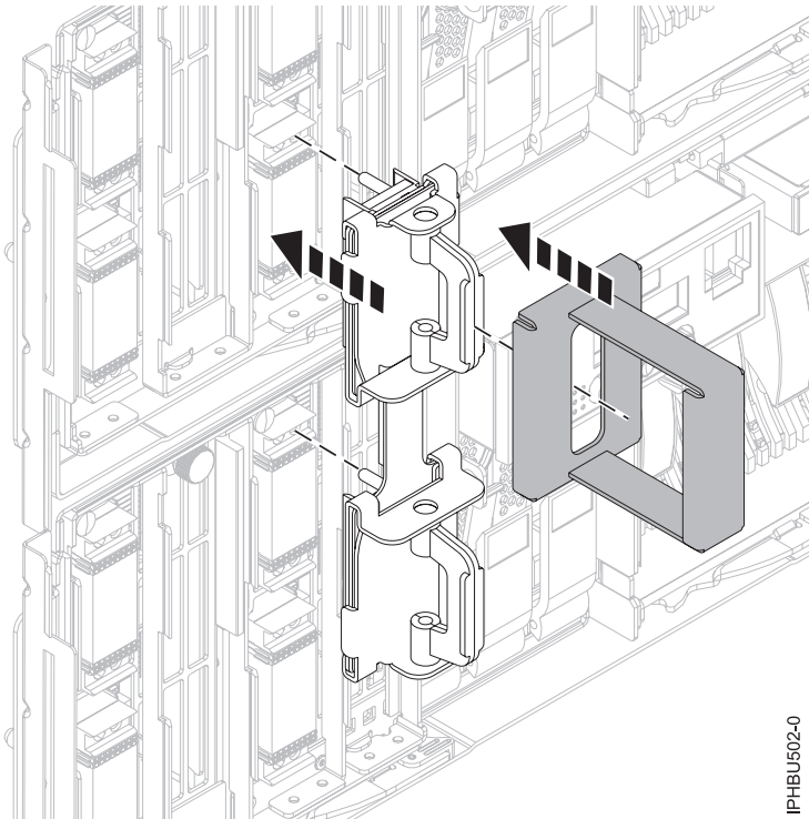
Figure 13. Utilisation de l'outil d'installation du câble SMP
