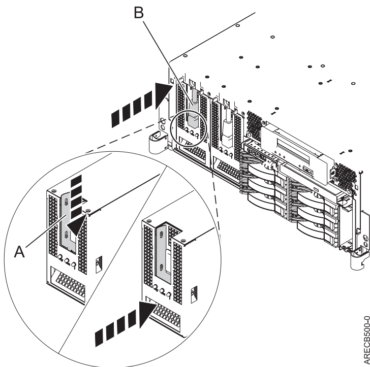
Figure 10. Remplacement d'une alimentation électrique
