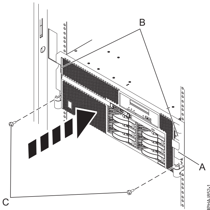
Figure 22. Installation du panneau avant d'un modèle monté en armoire
