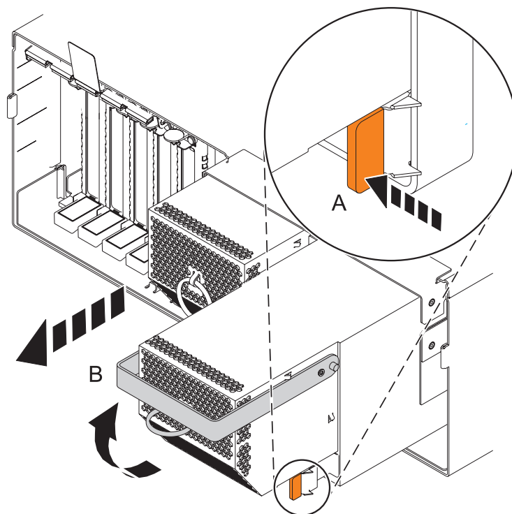
Figure 1. Alimentation électrique déverrouillée
