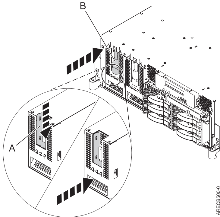
Figure 9. Remplacement d'une alimentation électrique
