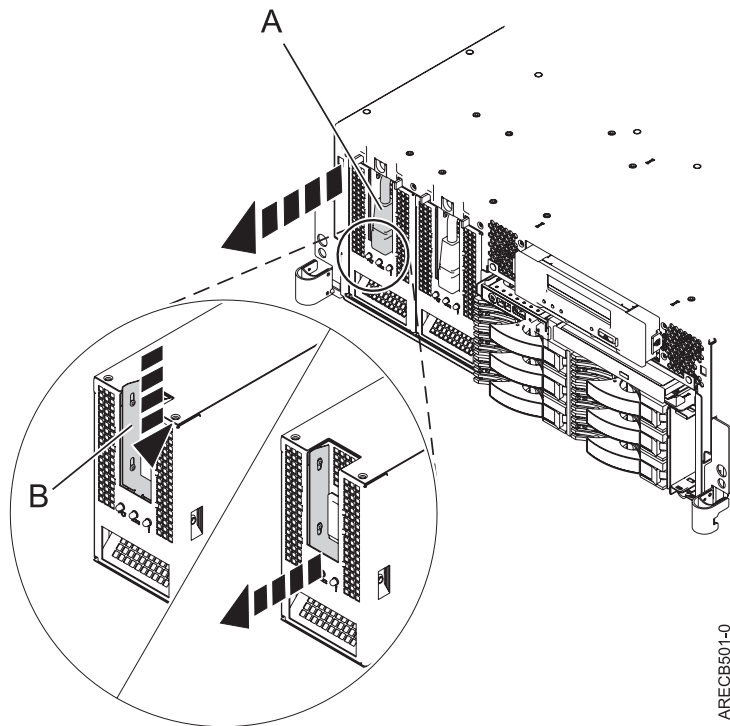
Figure 6. Retrait de l'alimentation électrique d'un modèle monté en armoire
