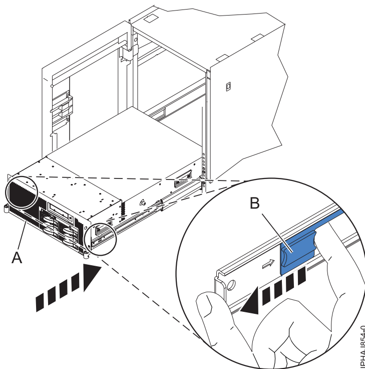
Figure 32. Libération des taquets de sécurité
