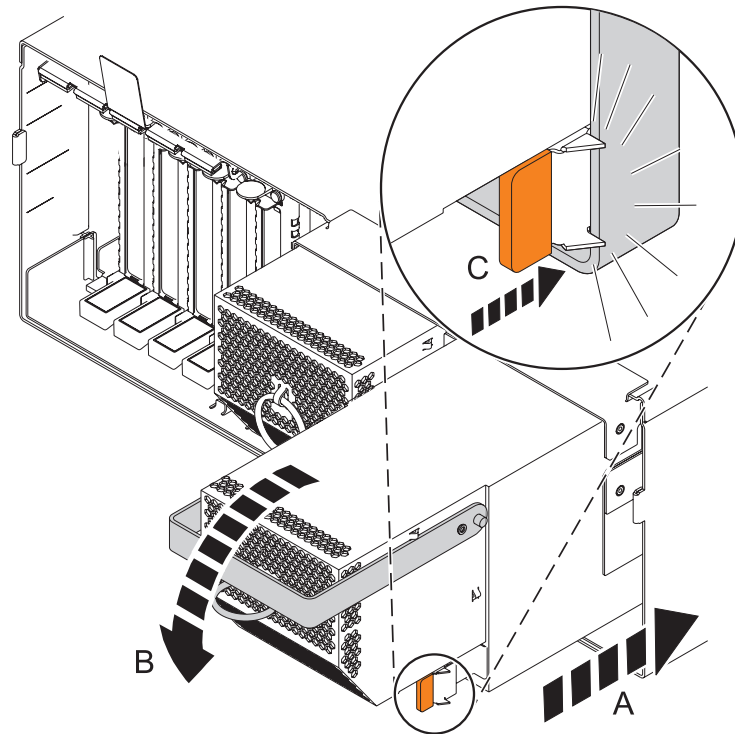
Figure 4. Remplacement de l'alimentation électrique
