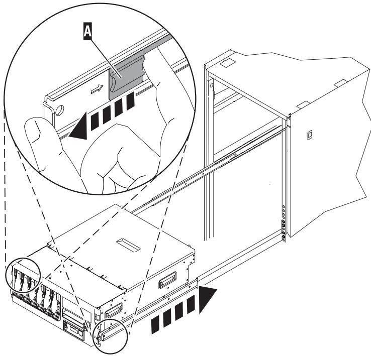
Figure 48. Libération des taquets de sécurité
