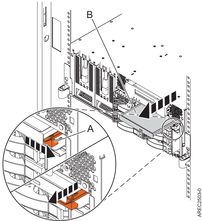
Figure 62. Retirez l'unité de stockage extra-plate Slimline
