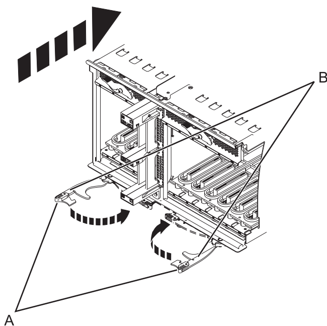
Figure 55. Installation de la carte d'entrée-sortie sur un modèle monté en armoire
