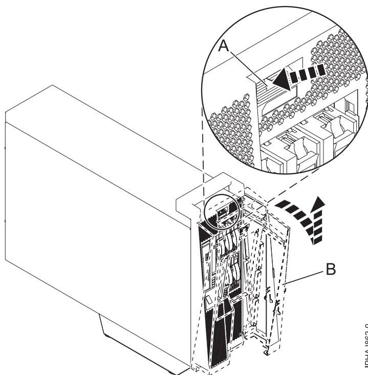
Figure 42. Rpetrait du volet
