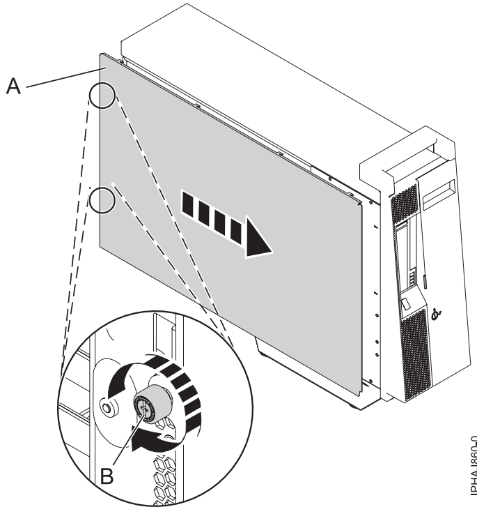
Figure 39. Installation du capot d'accès sur un modèle autonome
