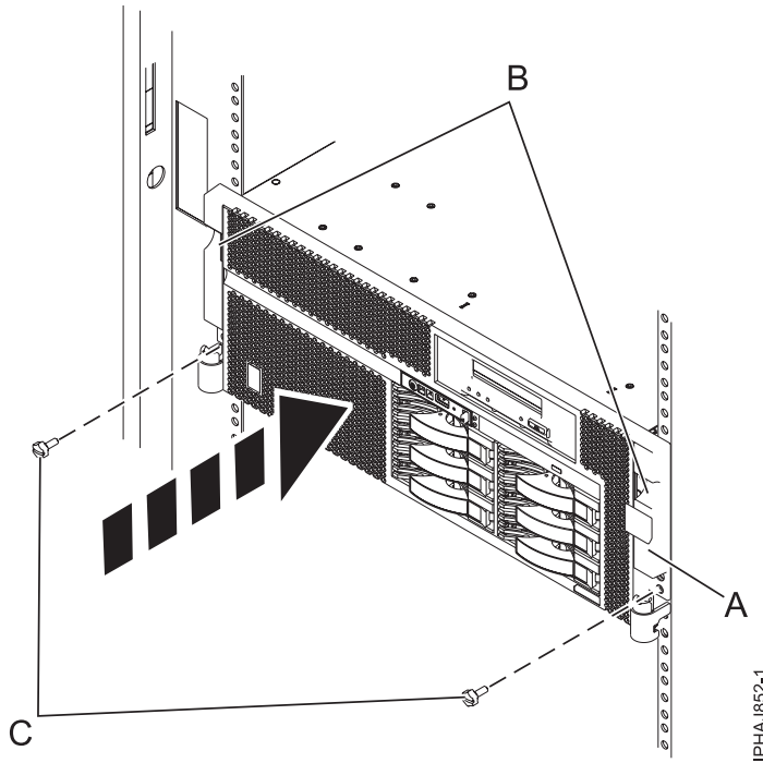
Figure 41. Installation du panneau avant d'un modèle monté en armoire
