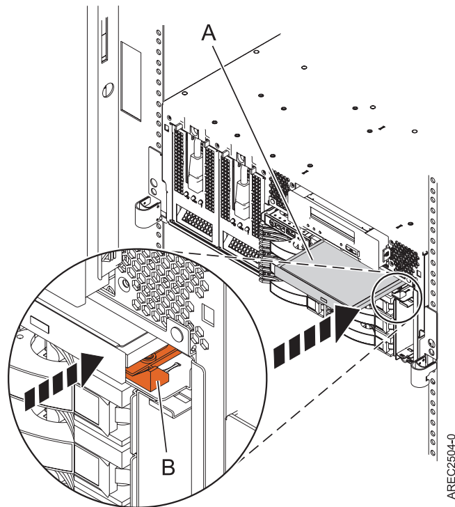
Figure 72. Installation d'une unité de stockage Slimline
