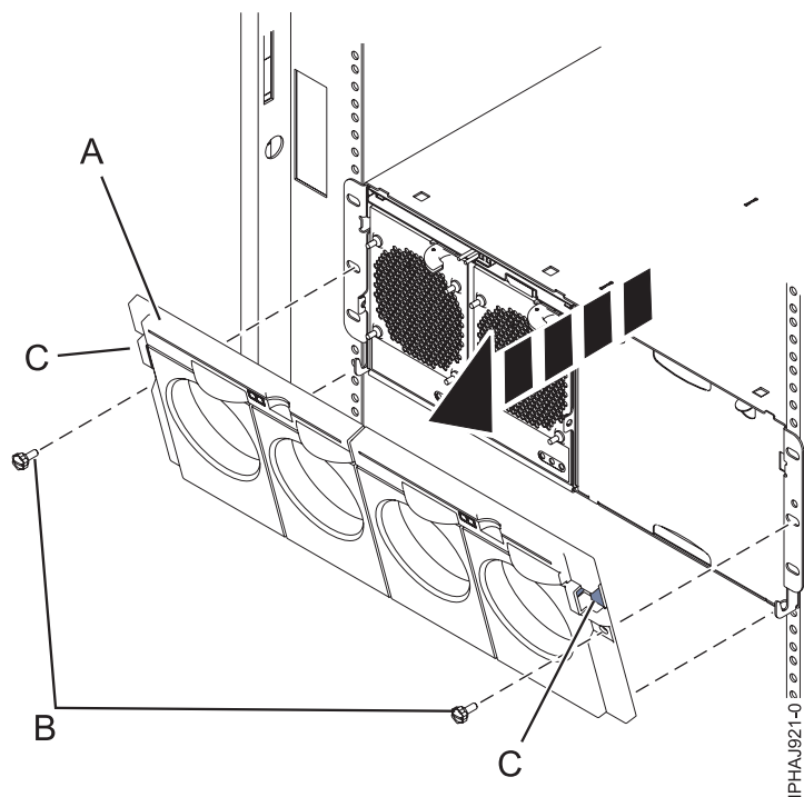
Figure 33. Retrait du panneau avant sur un modèle 14G/30
