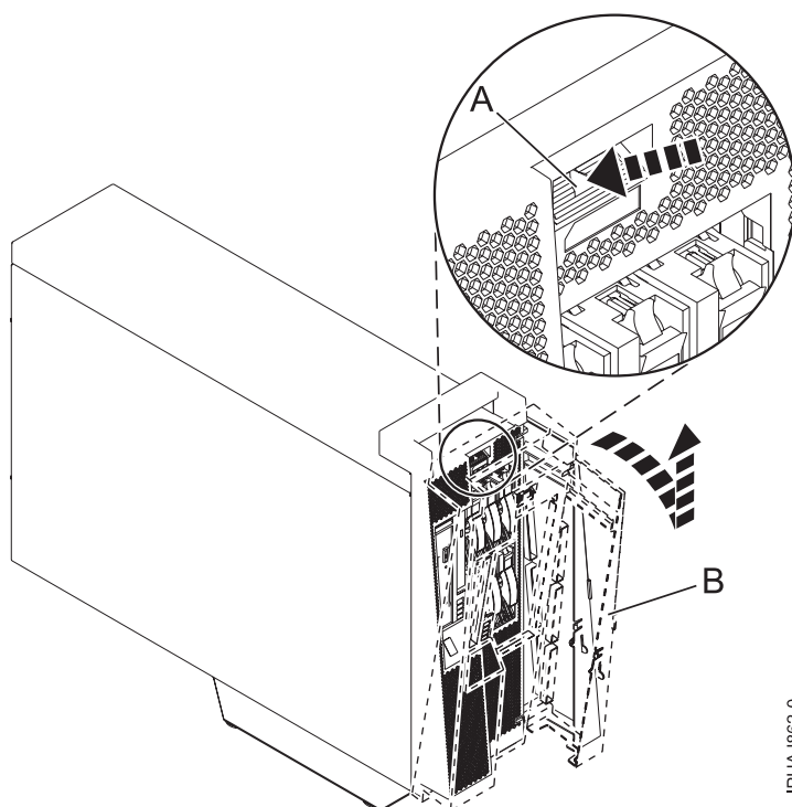
Figure 59. Retrait du volet
