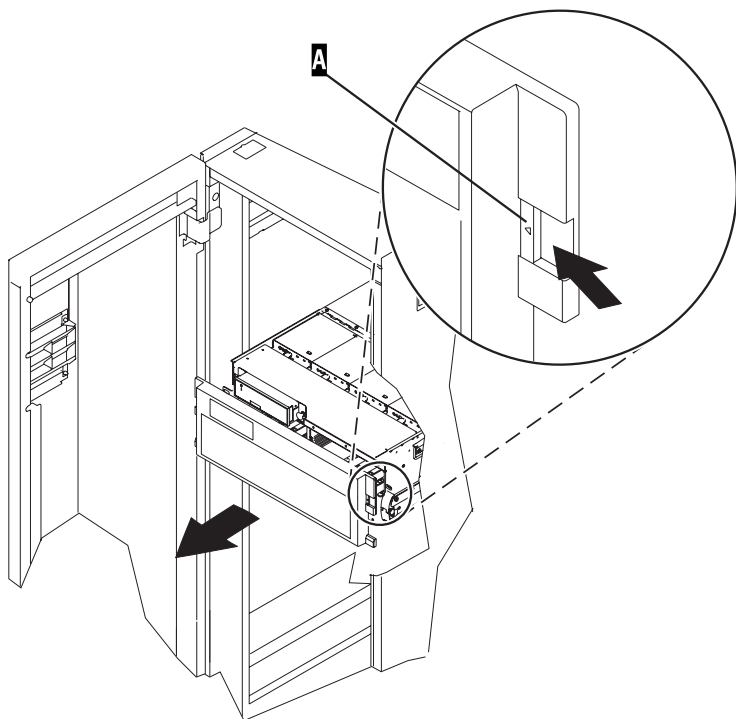
Figure 35. Retrait du panneau avant
