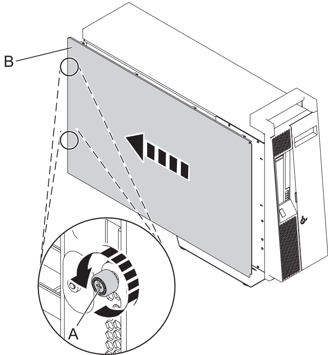
Figure 38. Retrait du capot d'accès d'un modèle autonome
