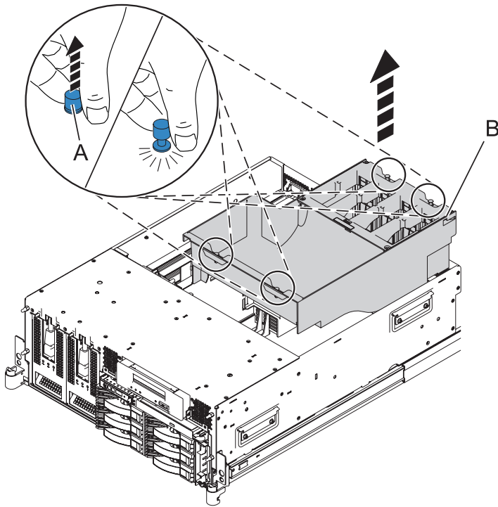
Figure 63. Retrait du capot de ventilation
