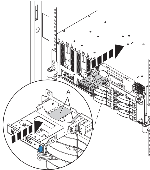
Figure 70. Remplacement du panneau de commande dans une unité centrale montée en armoire
