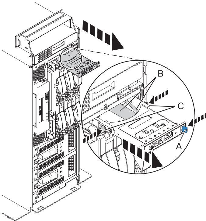
Figure 61. Retrait du panneau de commande d'une unité centrale autonome
