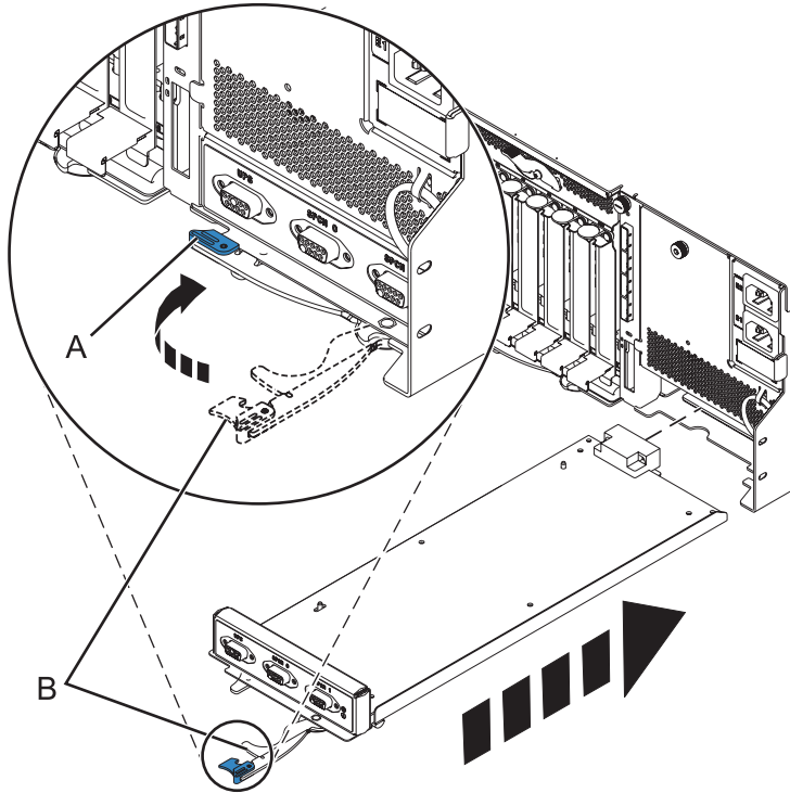
Figure 58. Remplacement de la carte EMC
