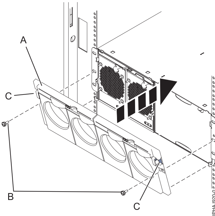
Figure 34. Panneau avant d'un modèle 14G/30
