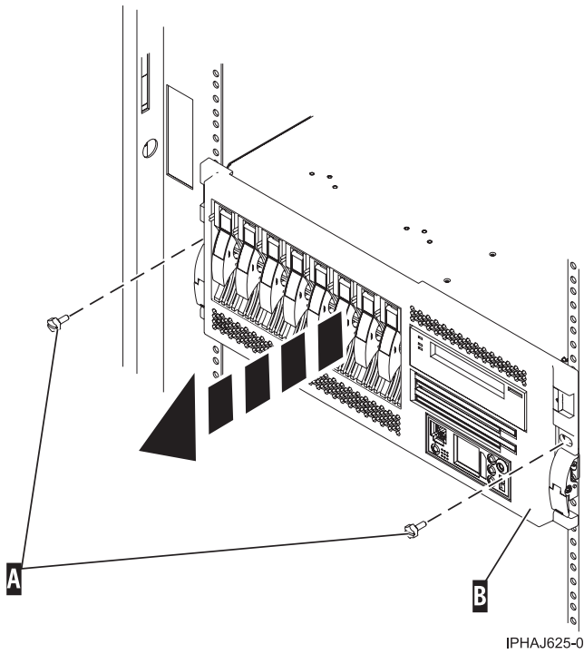
Figure 46. Retrait des vis moletées du système et de l'armoire
