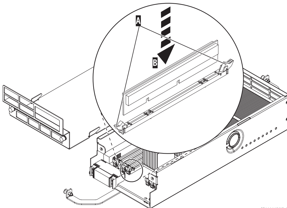
Figure 11. Remplacement d'un module de mémoire
