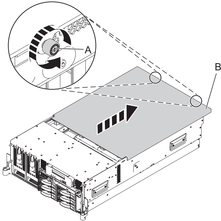
Figure 36. Retrait du capot d'accès d'un modèle monté en armoire
