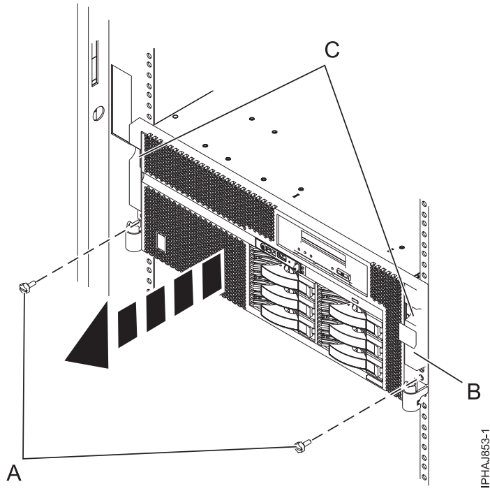
Figure 40. Retrait du panneau avant d'un modèle monté en armoire
