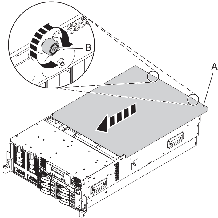
Figure 37. Installation du capot d'accès du modèle monté en armoire
