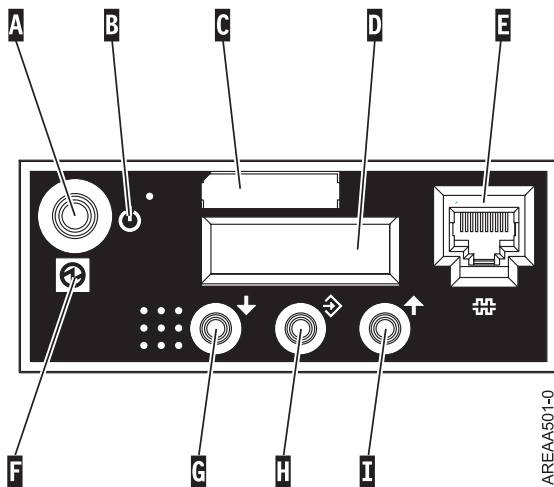
Figure 30. Panneau de commande du modèle 5/70
