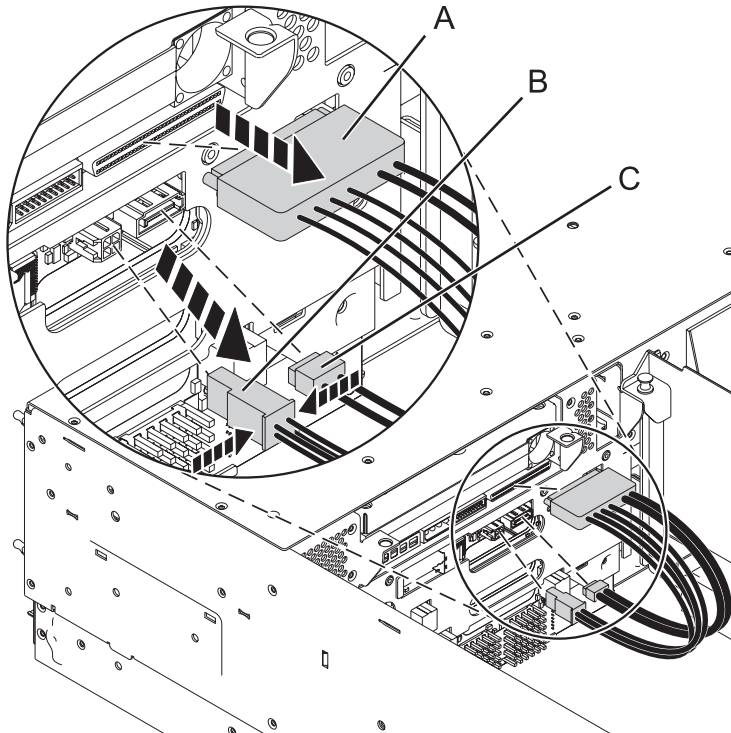
Figure 64. Déconnexion des câbles de l'unité de stockage
