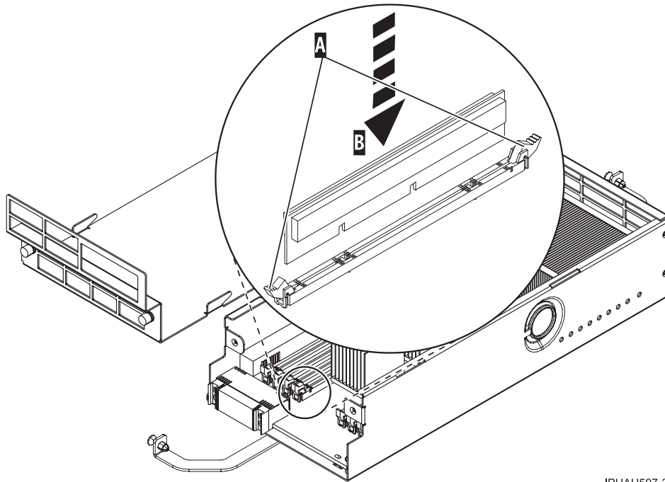
Figure 4. Remplacement d'un module de mémoire
