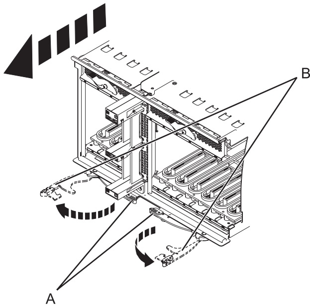
Figure 56. Retrait de la carte d'entrée-sortie
