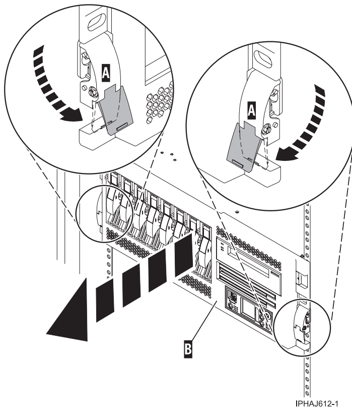
Figure 47. Libération des loquets de sécurité
