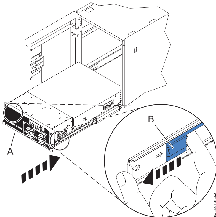
Figure 51. Déblocage des taquets de sécurité du rail
