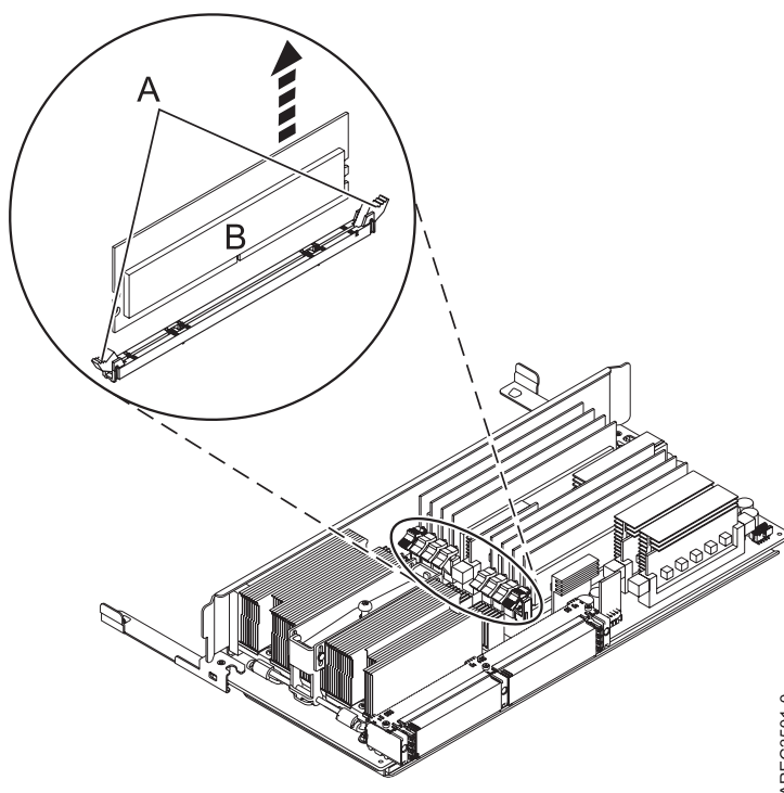
Figure 28. Retrait d'un module de mémoire
