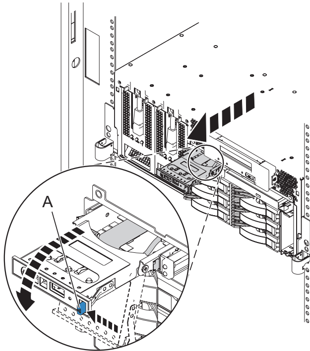
Figure 53. Ouverture du panneau de commande
