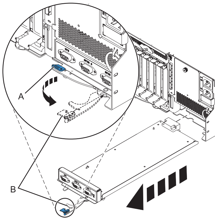
Figure 57. Retrait de la carte EMC du système
