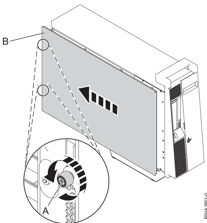
Figure 60. Retrait du capot d'accès d'un modèle autonome
