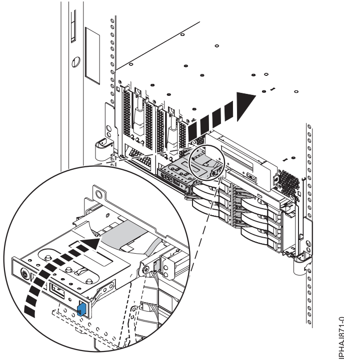
Figure 54. Remplacez le panneau de commande dans le boîtier
