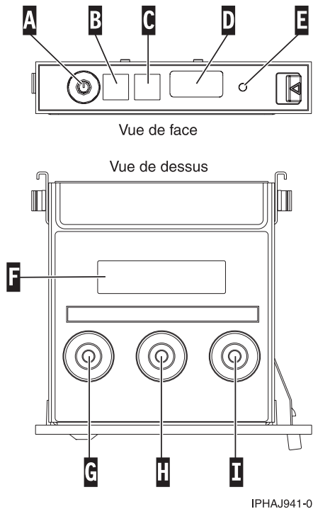
Figure 17. Panneau de commande des modèles 03E/4A, 04E/8A.
