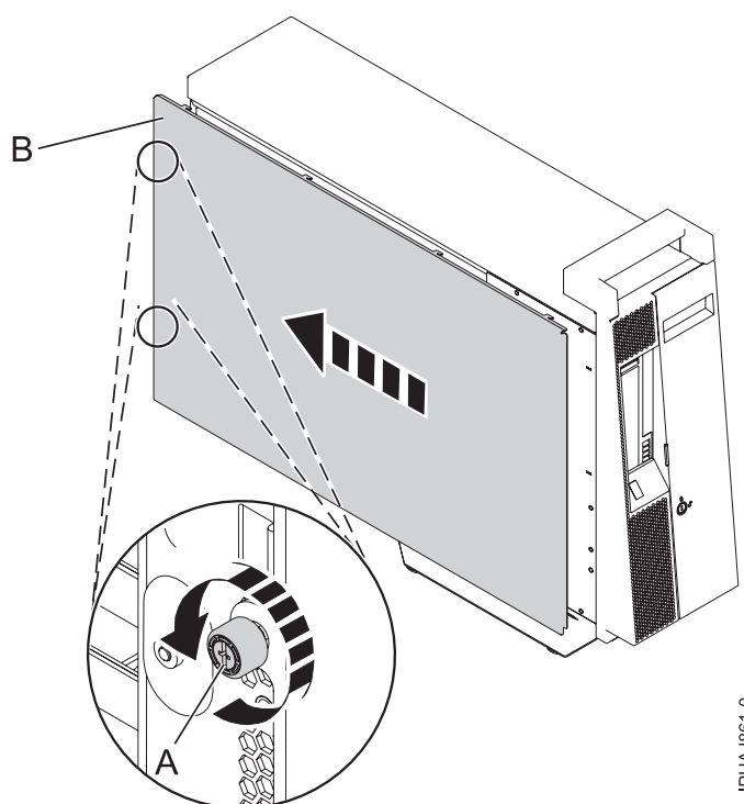
Figure 24. Retrait du capot d'accès d'un modèle autonome
