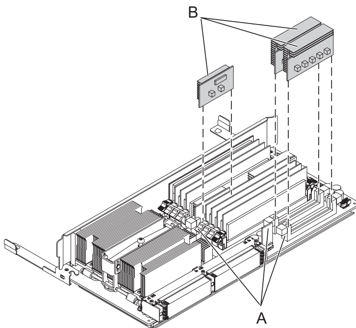
Figure 7. Régulateurs de tension (B) illustrés au-dessus des emplacements de régulateur de tension du bloc processeur système (A)
