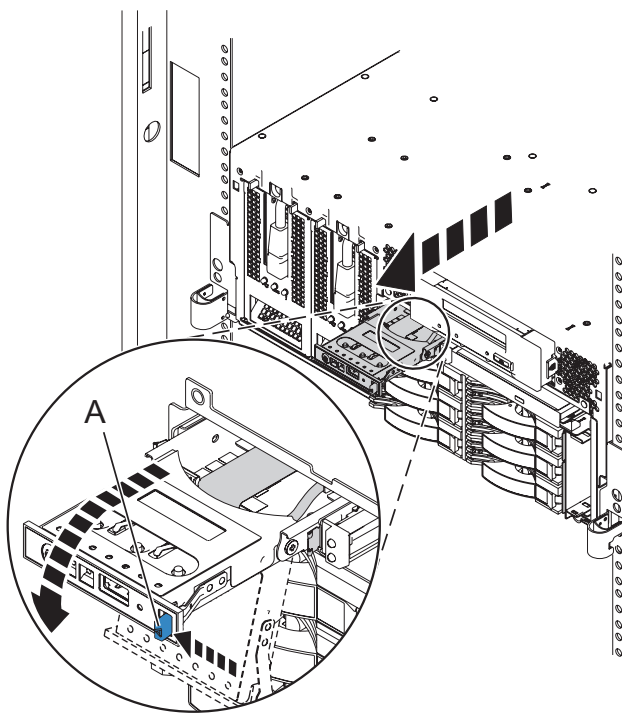
Figure 39. Ouverture du panneau de commande
