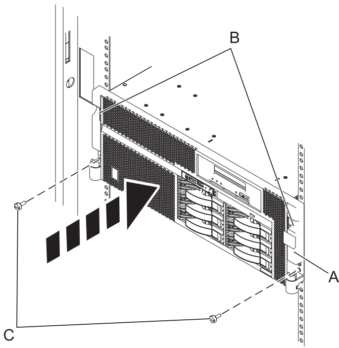
Figure 35. Mise en place du système dans l'armoire et fixation des vis moletées
