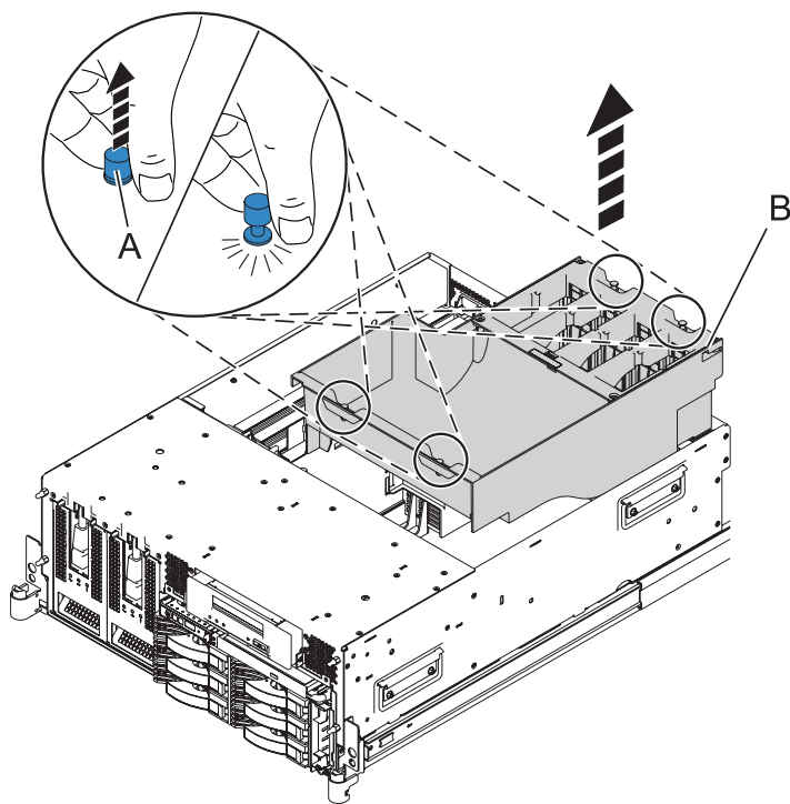
Figure 48. Retrait du capot de ventilation
