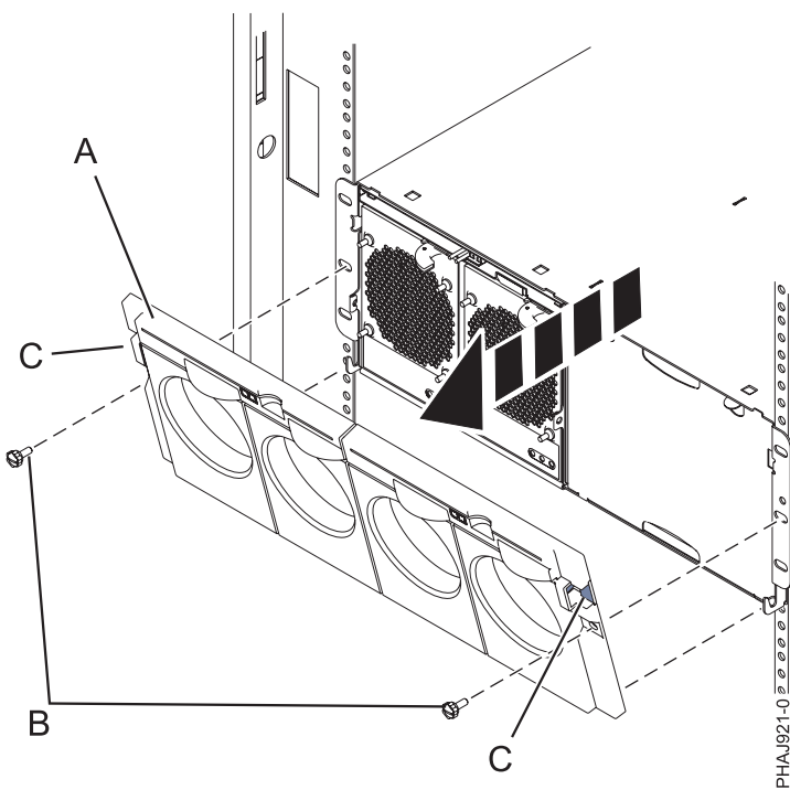
Figure 19. Retrait du panneau avant sur un modèle 14G/30
