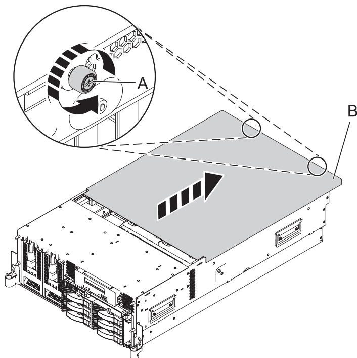
Figure 22. Retrait du capot d'accès d'un modèle monté en armoire
