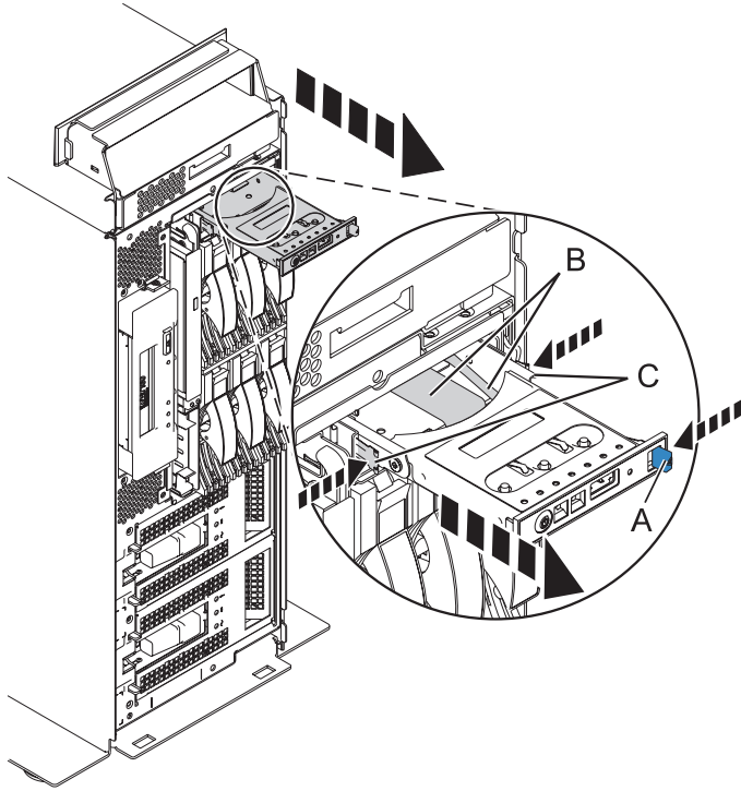
Figure 46. Retrait du panneau de commande d'une unité centrale autonome
