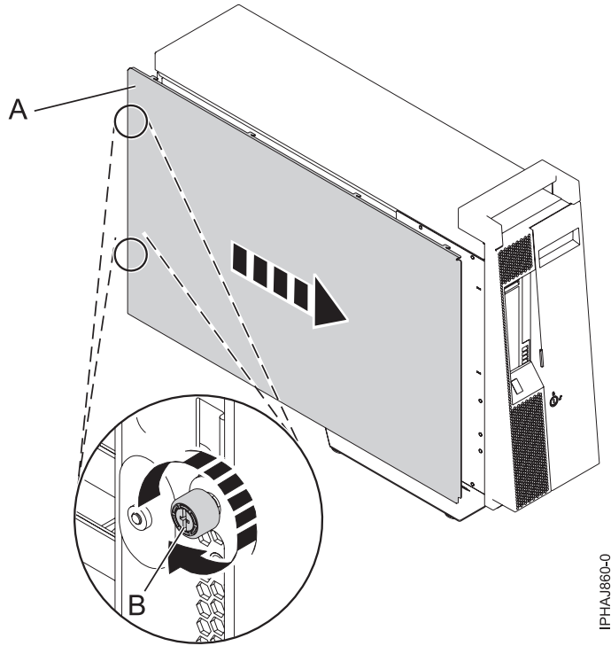
Figure 25. Installation du capot d'accès sur un modèle autonome
