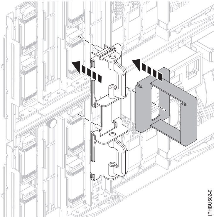
Figure 18. Utilisation de l'outil de câblage SMP
