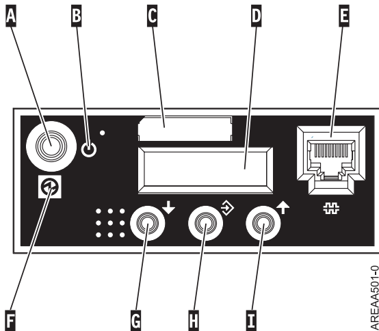
Figure 16. Panneau de commande du modèle 5/70
