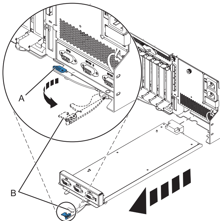
Figure 43. Retrait de la carte EMC du système
