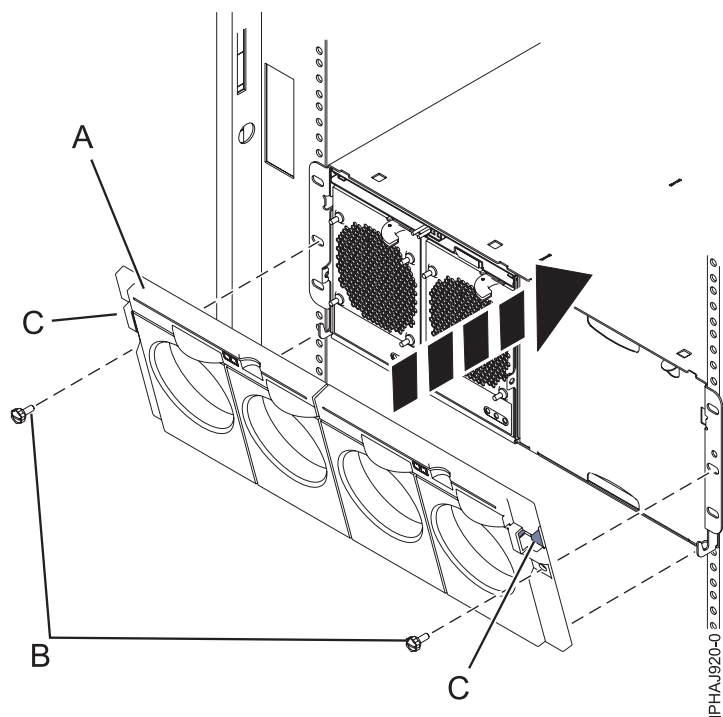
Figure 20. Panneau avant d'un modèle 14G/30
