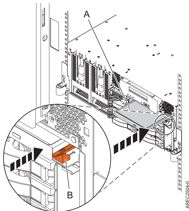
Figure 57. Installation d'une unité de stockage Slimline
