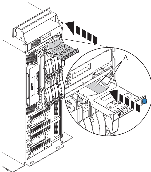
Figure 56. Remplacement du panneau de commande dans une unité centrale autonome
