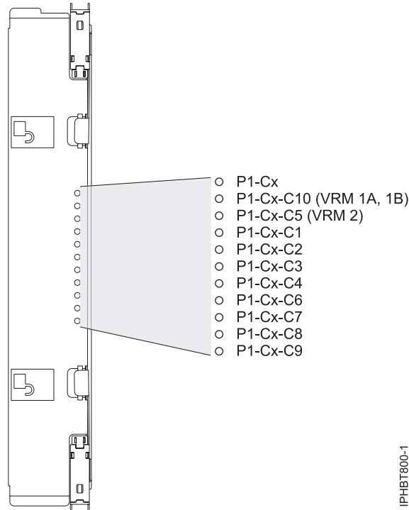
Figure 3. Voyants d'identification des régulateurs de tension VRM 1A, 1B et VRM 2 et codes d'emplacement
