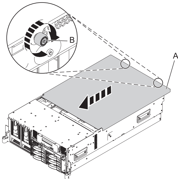
Figure 23. Installation du capot d'accès du modèle monté en armoire
