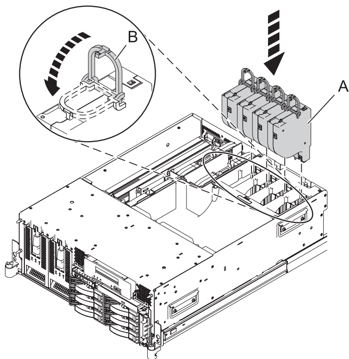
Figure 12. Remplacement des ventilateurs
