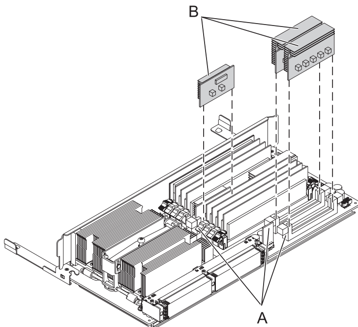
Figure 5. Régulateurs de tension (B) illustrés au-dessus des emplacements de régulateur de tension du bloc processeur système (A)
