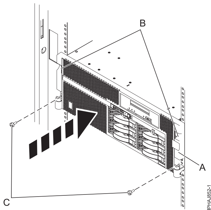
Figure 27. Installation du panneau avant sur un modèle monté en armoire
