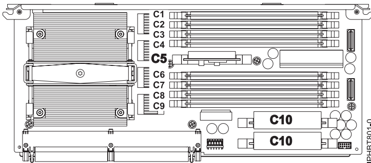
Figure 4. Emplacements de régulateur de tension C5 (VRM 2) et C10 (VRM 1A, 1B)
