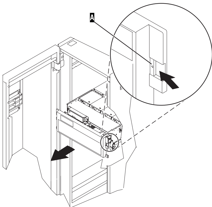
Figure 21. Retrait du panneau avant
