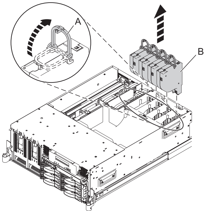
Figure 13. Retrait du ventilateur pour les systèmes 03E/4A, 07M/15 et
