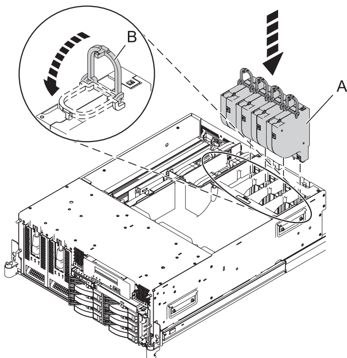
Figure 15. Remplacement du ventilateur pour les systèmes 03E/4A, 07M/15 et
