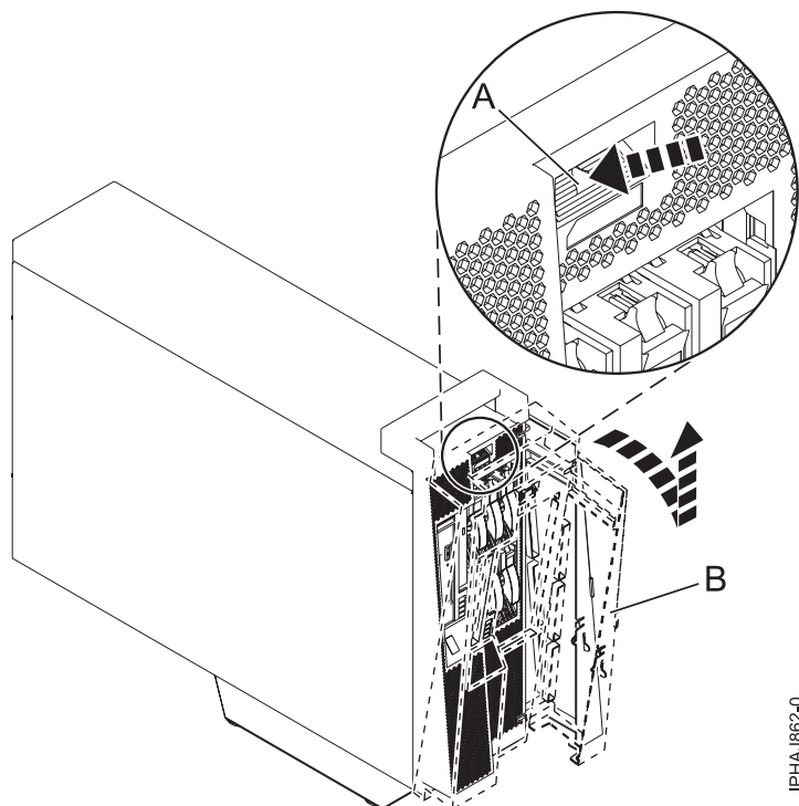
Figure 28. Retrait du volet
