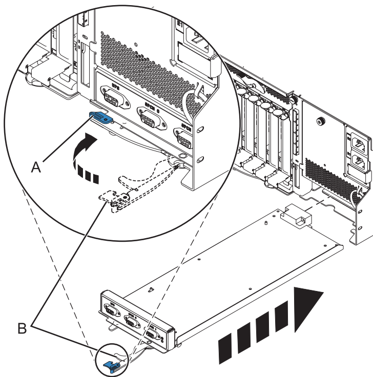
Figure 44. Remplacement de la carte EMC
