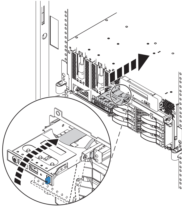
Figure 40. Remplacez le panneau de commande dans le boîtier
