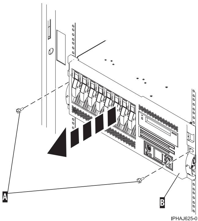
Figure 32. Retrait des vis moletées du système et de l'armoire
