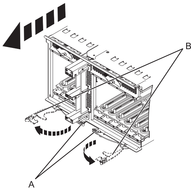
Figure 42. Retrait de la carte d'entrée-sortie
