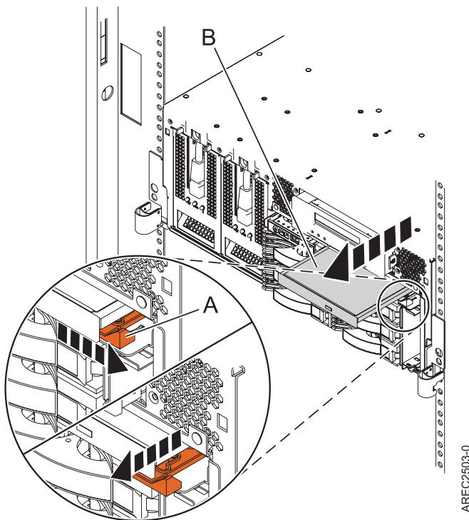
Figure 47. Retirez l'unité de stockage extra-plate Slimline
