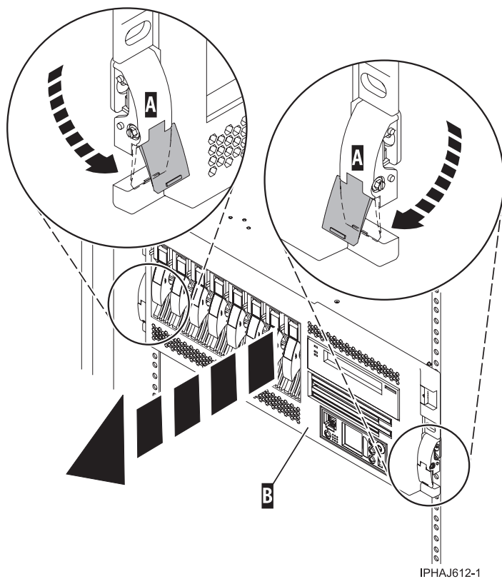
Figure 33. Libération des loquets de sécurité
