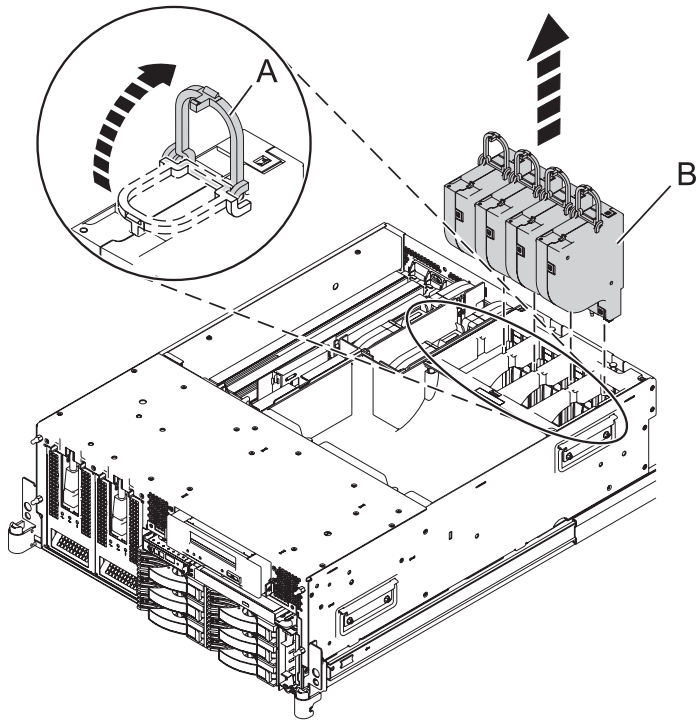
Figure 11. Retrait du ventilateur pour les systèmes 03E/4A, 07M/15 et
