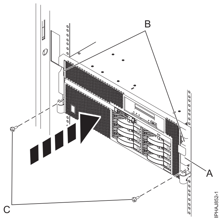
Figure 38. Remise en place des vis moletées
