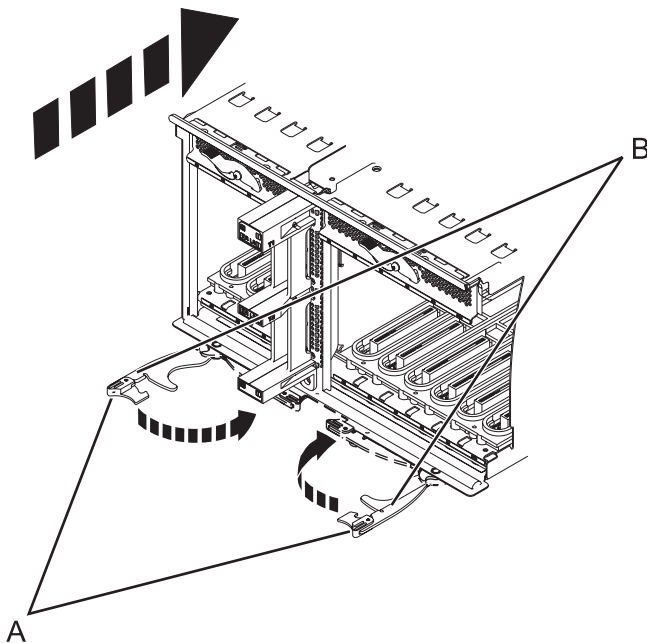
Figure 41. Installation de la carte d'entrée-sortie sur un modèle monté en armoire
