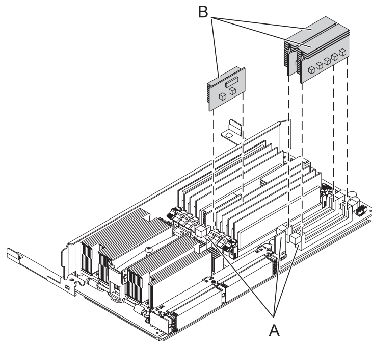
Figure 2. Régulateurs de tension (B) (1,5 V cc et 2,5 V cc) affichés avec leurs emplacements (A).
