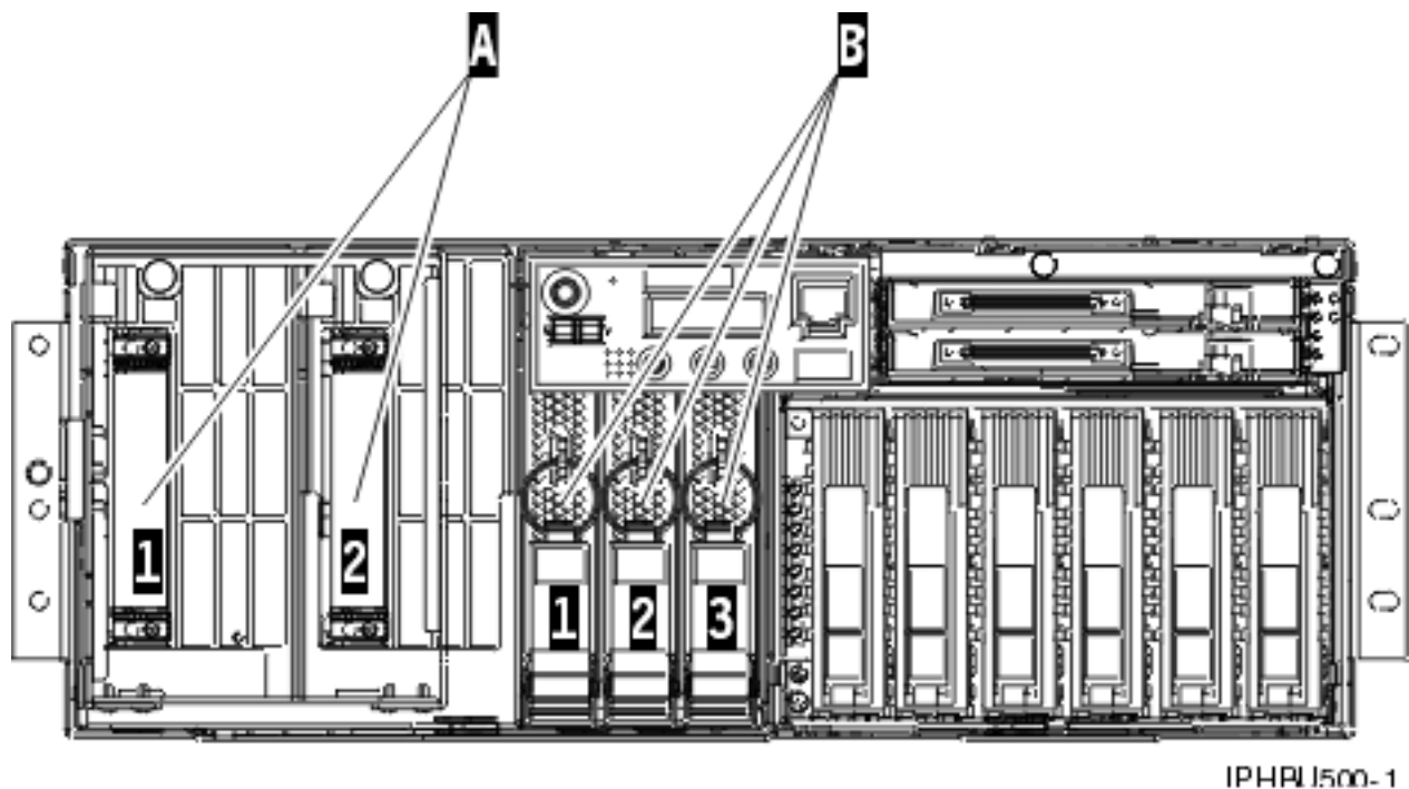
Figure 1. Blocs processeurs système et blocs régulateurs de tension (vue de face)
