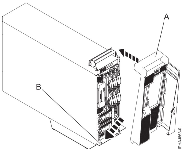
Figure 29. Remplacement du panneau du modèle
