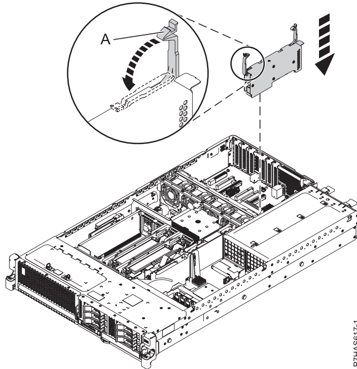
Figure 2. Installation de l'adaptateur FC EJ0H sur un système
