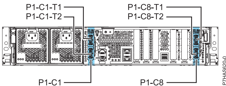
Figure 1. Emplacements et codes d'emplacement d'adaptateur GX
