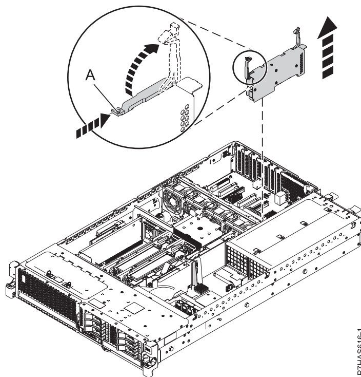
Figure 5. Retrait d'un adaptateur d'un système
