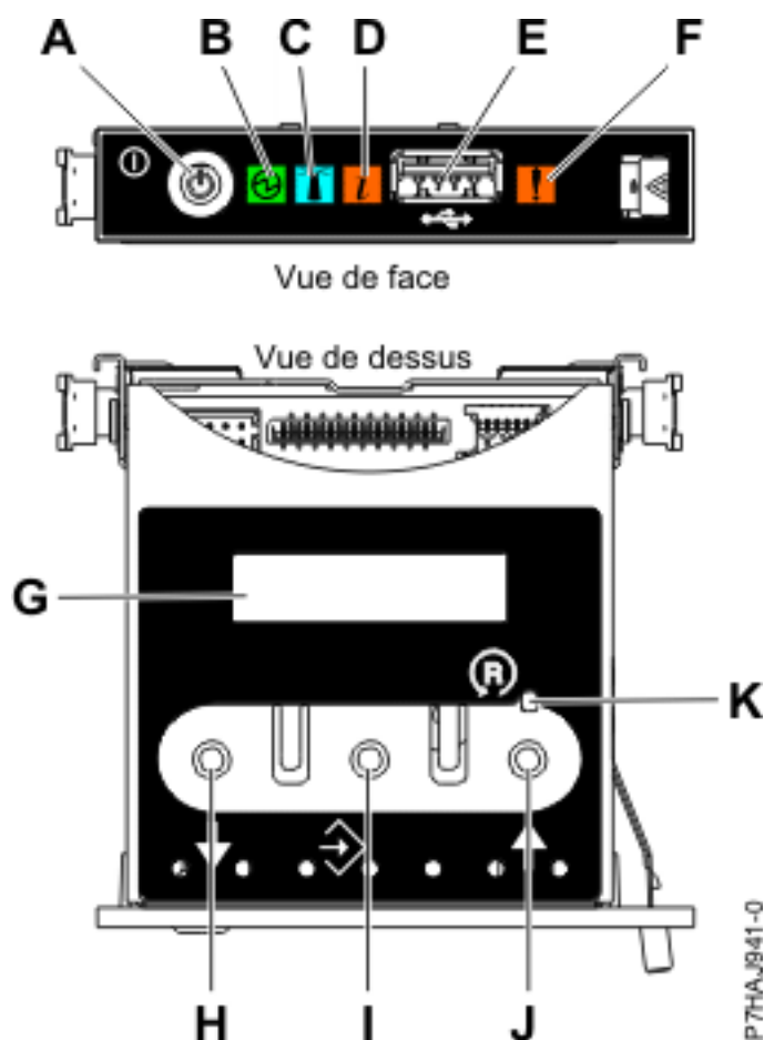
Figure 9. Panneau de commande
