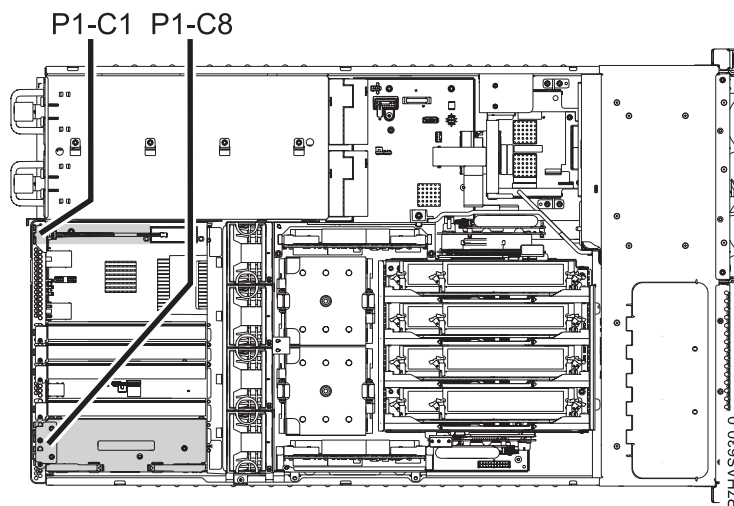
Figure 4. Emplacements de l'adaptateur GX
