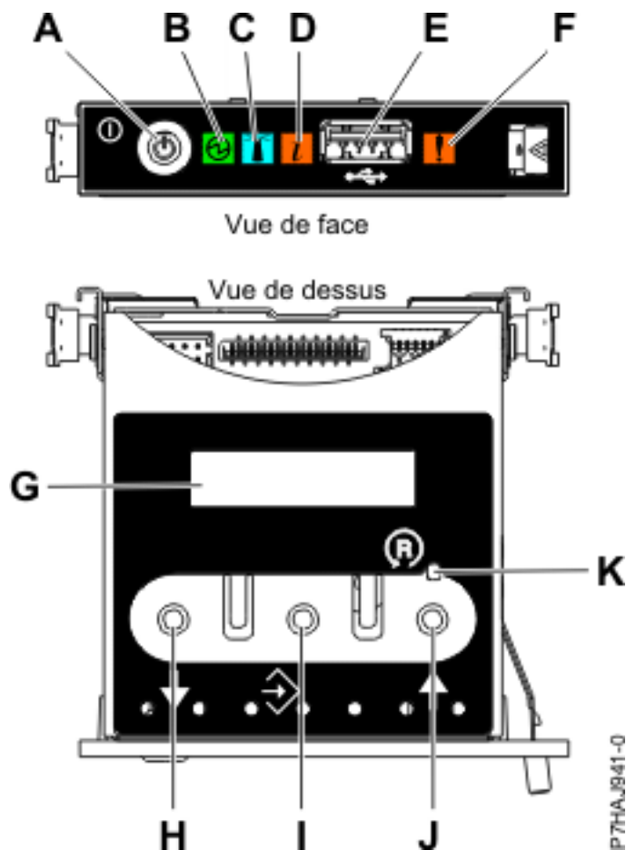
Figure 8. Panneau de commande
