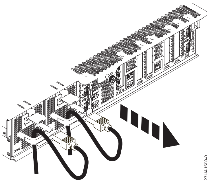
Figure 15. Retrait des cordons d'alimentation
