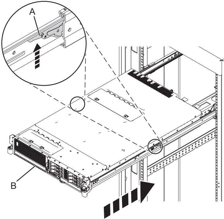
Figure 17. Déverrouillage des taquets de sécurité des glissières
