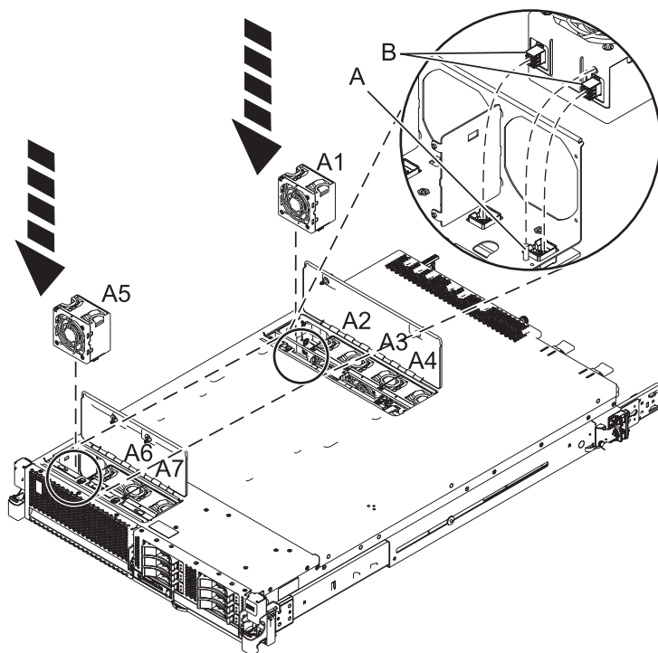
Figure 2. Remise en place du ventilateur dans un modèle 31E/2B, 31E/1C, 31E/1D, 31E/2C ou 31E/2D monté en armoire
