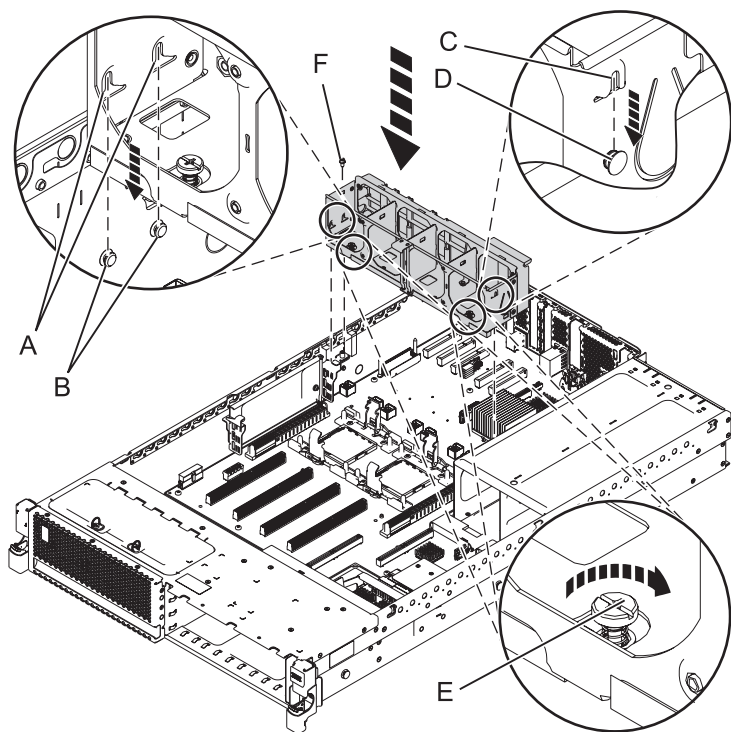
Figure 10. Remise en place du boîtier du ventilateur intermédiaire du modèle 31E/2B, 31E/1C, 31E/1D, 31E/2C ou 31E/2D
