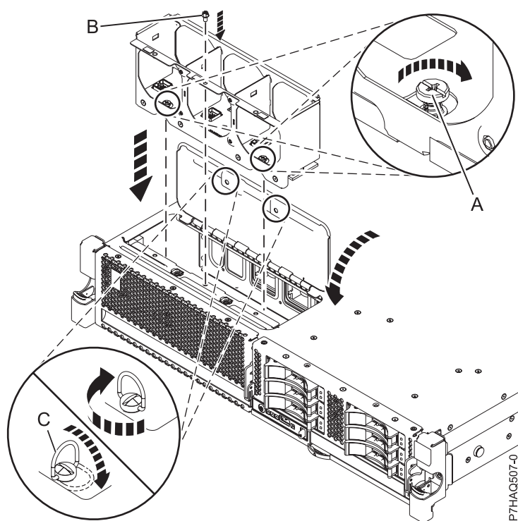
Figure 5. Remise en place du boîtier du ventilateur avant sur le système 31E/2B, 31E/1C, 31E/1D, 31E/2C ou 31E/2D
