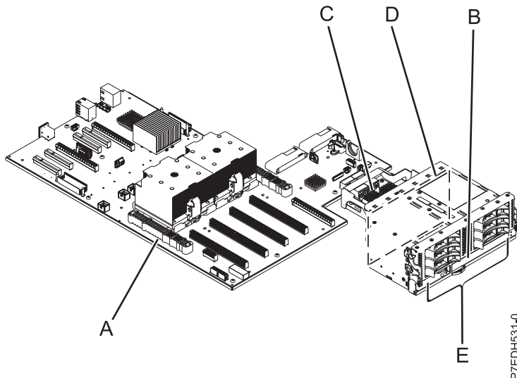
Figure 1. Présentation du sous-système SAS de base
