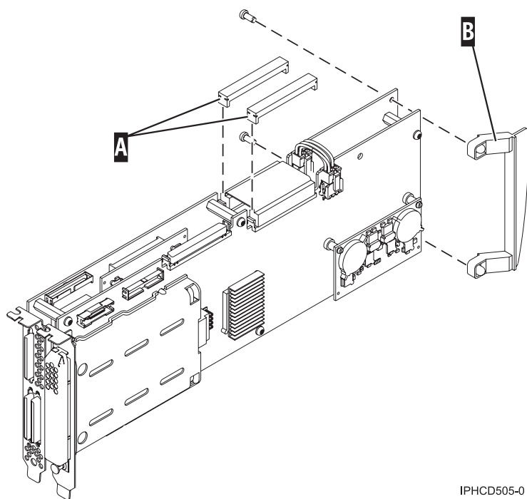
Figure 81. Préparation de la carte pour être placée dans une cassette
