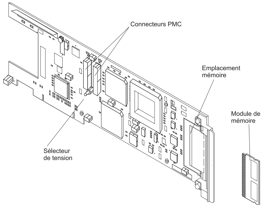
Figure 82. Carte PCI de base ARTIC960Hx
