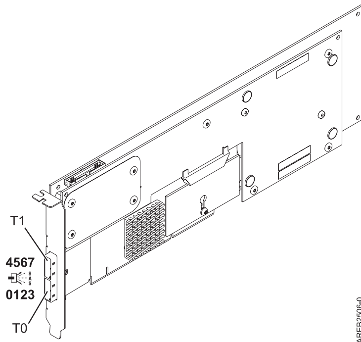
Figure 69. carte SAS RAID PCI-X DDR double accès -x4
