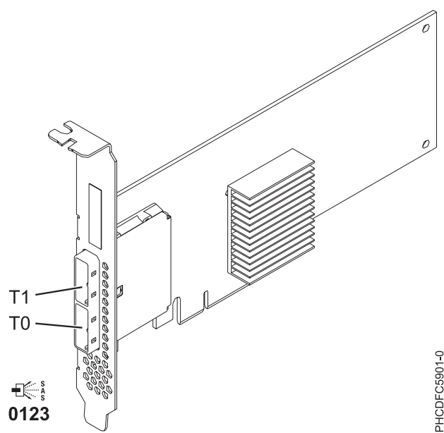
Figure 65. Carte PCIe SAS double accès x4
