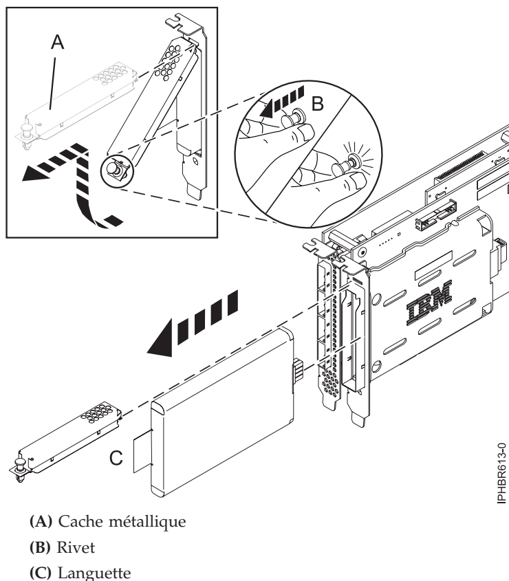
Figure 87. Remplacement de la batterie du cache d'une carte 572F/575C
