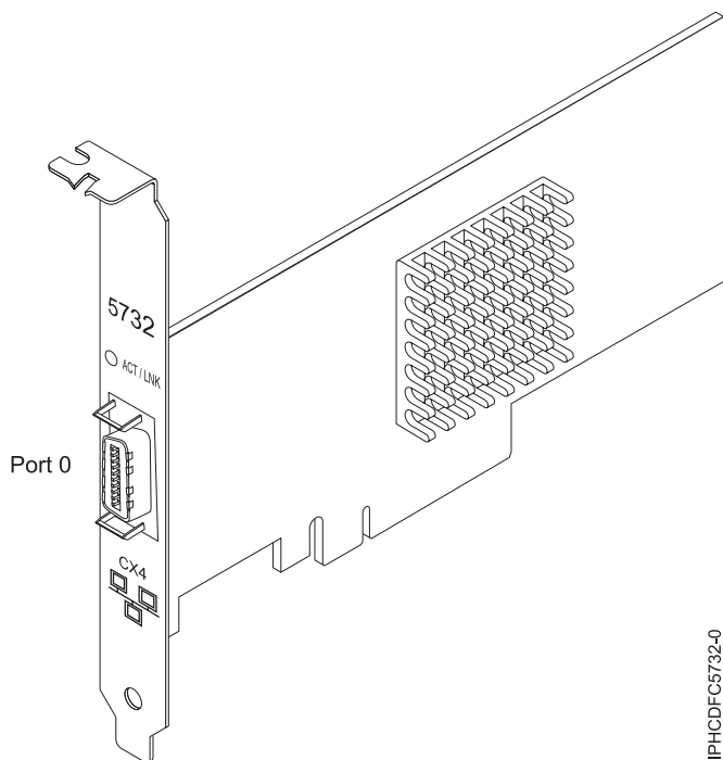
Figure 45. carte PCI Express (PCIe) 10 Gigabit Ethernet-CX4
