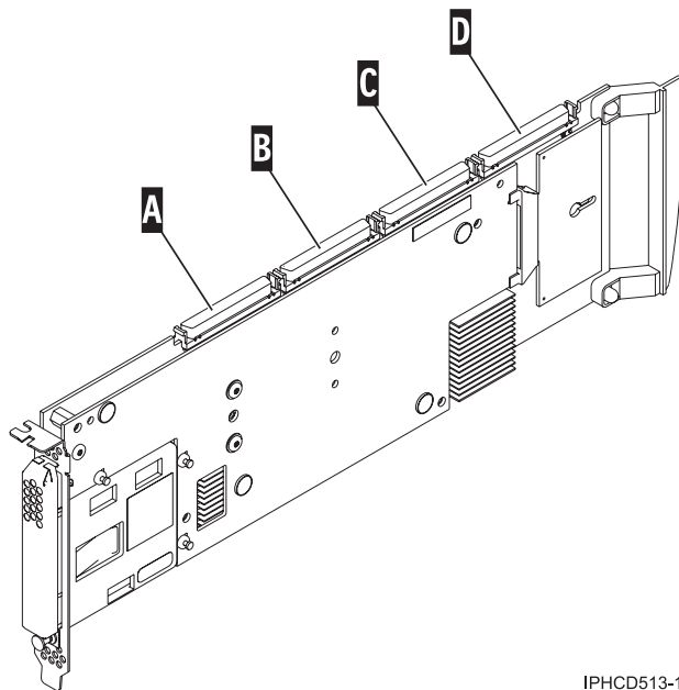
Figure 79. Connecteurs SCSI de la carte
