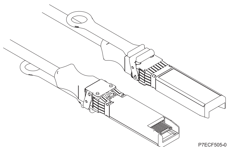
Figure 57. Schéma des extrémités du câble
