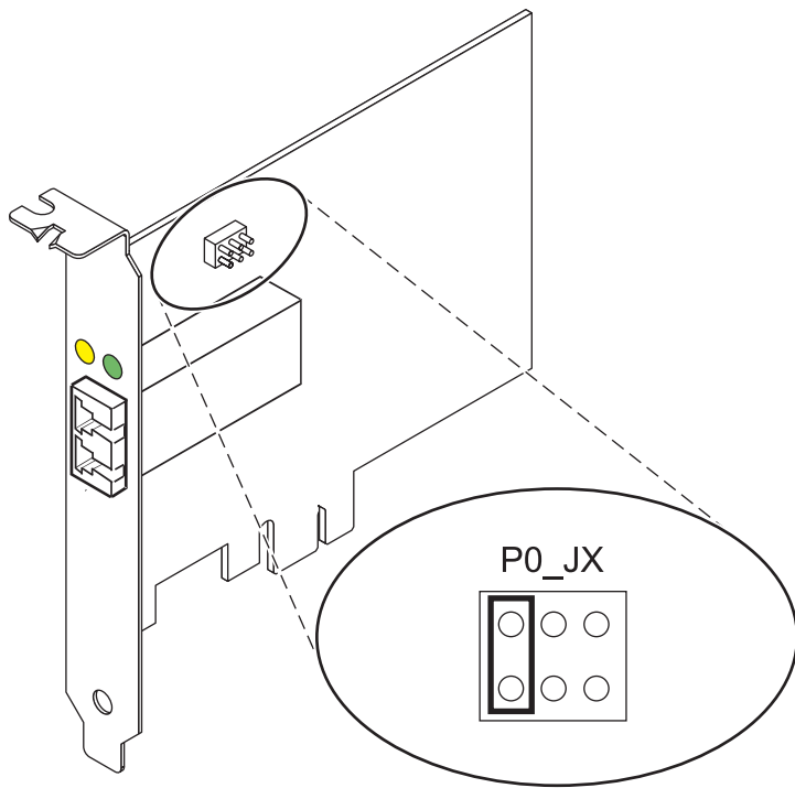
Figure 16. Cavalier ID unité
