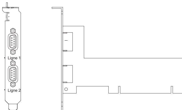
Figure 7. Carte PCI à deux ports asynchrones EIA-232
