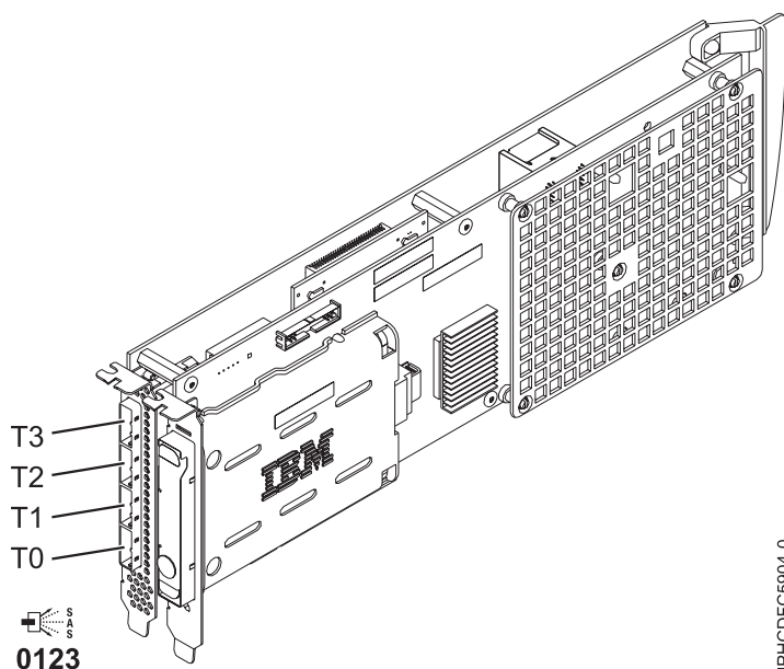
Figure 71. Carte SAS RAID PCI-X DDR 1,5 Go de cache
