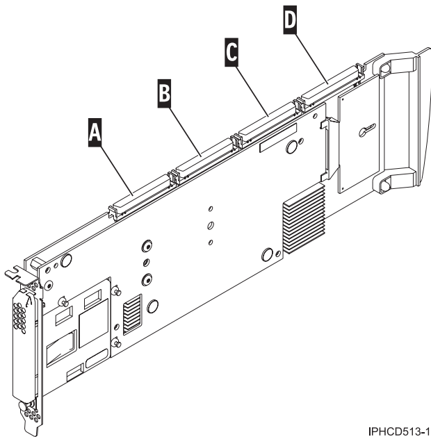
Figure 76. Connecteurs SCSI de la carte
