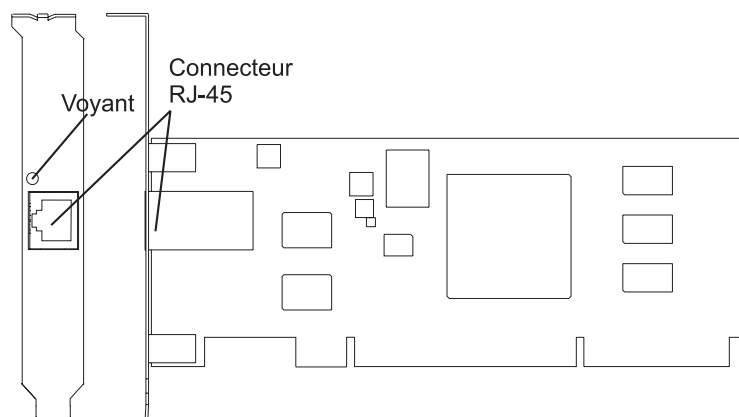
Figure 26. Carte PCI-X TOE iSCSI TX 1 Gbit
