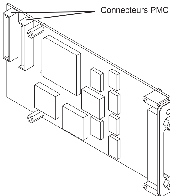
Figure 83. Carte PMC 4 ports sélectionnables
