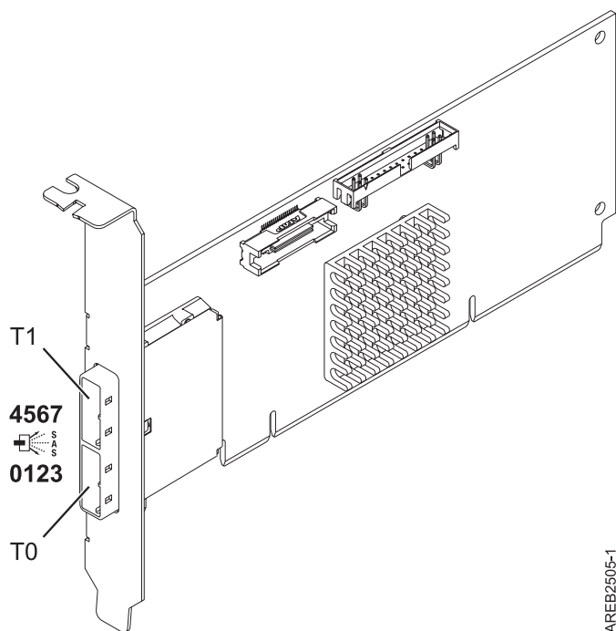
Figure 72. Carte SAS PCI-X DDR externe double accès – x4
