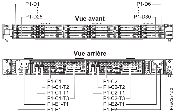
Figure 84. Codes d'emplacement de la carte PCIe2 SAS RAID intégrée avec cache de 3,1 Go
