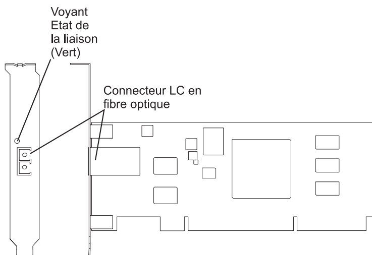
Figure 25. Carte PCI-X TOE iSCSI SX 1 Gbit
