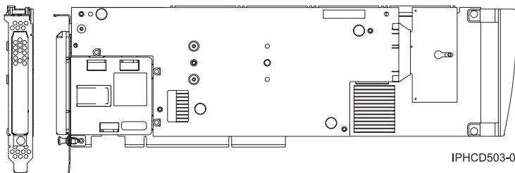
Figure 75. Vue latérale et vue d'extrémité de la carte
