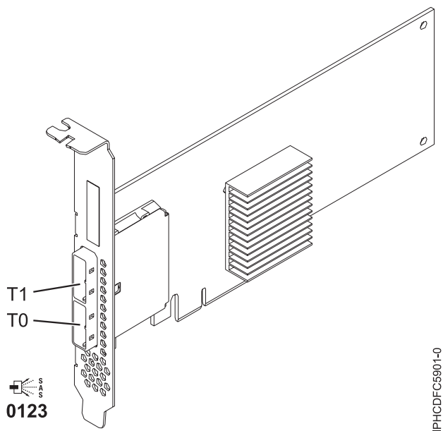
Figure 68. Carte PCIe SAS double accès x4
