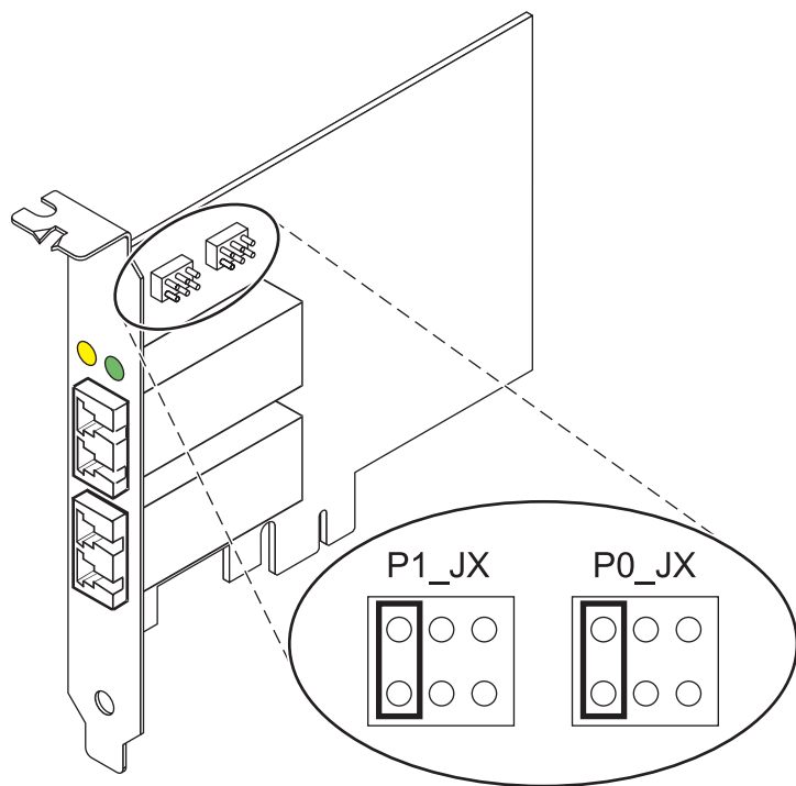
Figure 18. Cavalier ID unité
