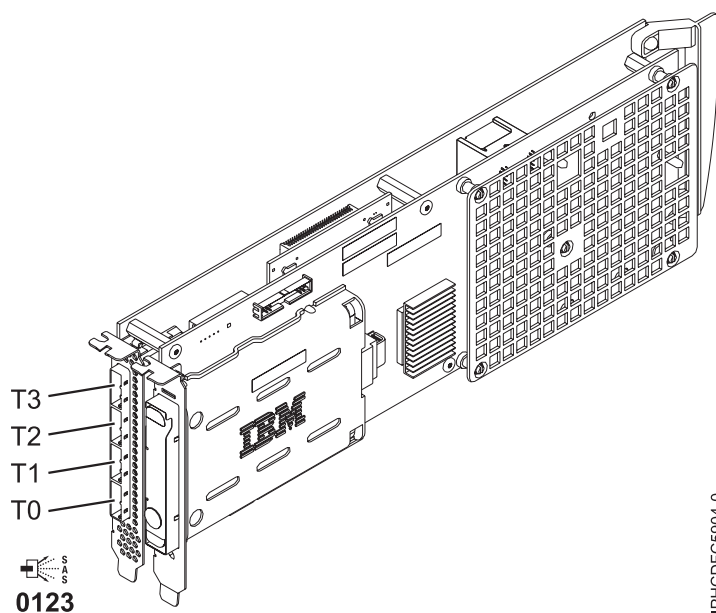
Figure 70. Carte SAS RAID PCI-X DDR 1,5 Go de cache
