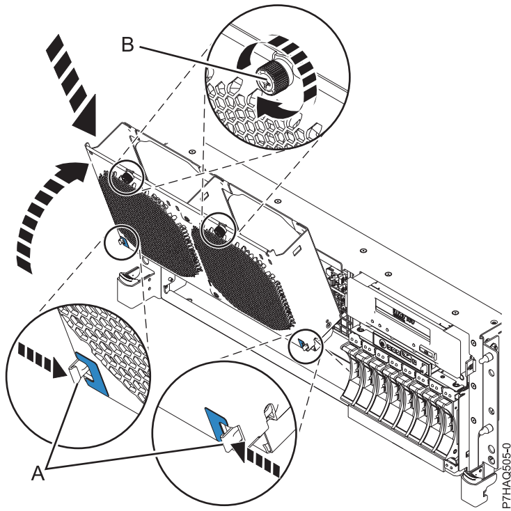
Figure 5. Remise en place du boîtier de ventilation sur le modèle 02E/4B, 02E/4C, 02E/4D, 05F/6B, 05E/6C ou 05E/6D
