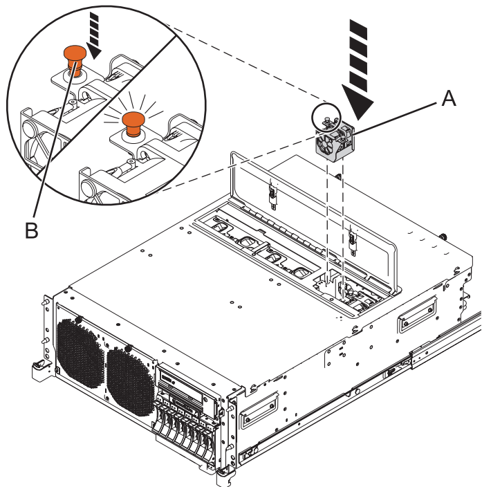
Figure 12. Installation d'un ventilateur dans l'02E/4B, 02E/4C, 02E/4D, 05F/6B, 05E/6C ou 05E/6D
