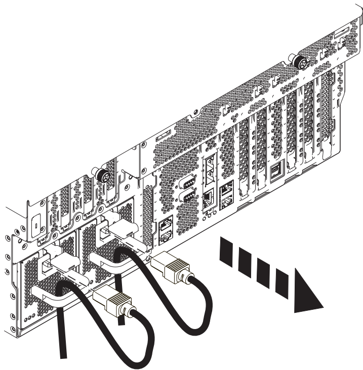
Figure 30. Retrait des cordons d'alimentation pour un système monté en armoire
