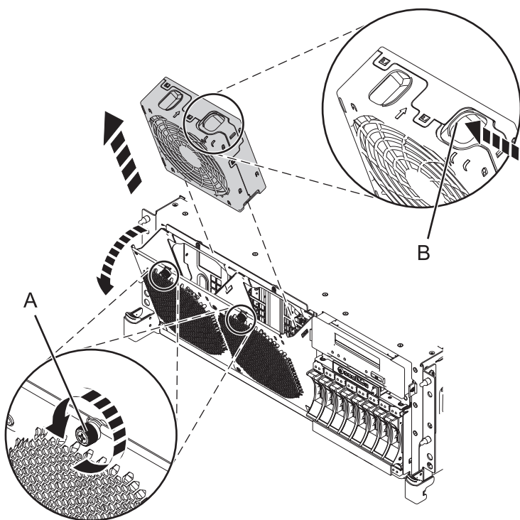
Figure 1. Retrait d'un ventilateur du modèle 02E/4B, 02E/4C, 02E/4D, 05F/6B, 05E/6C ou 05E/6D
