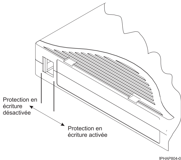
Figure 3. Positionnement du taquet de protection contre l'écriture
