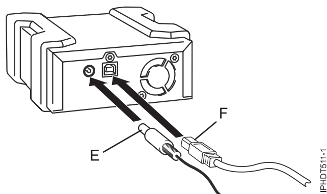
Figure 12. Unité externe, vue arrière et connecteurs
