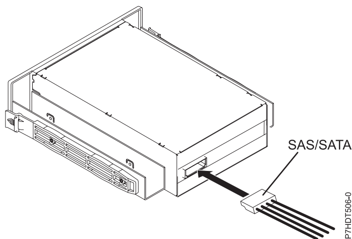
Figure 14. Unité interne, vue arrière et connecteur
