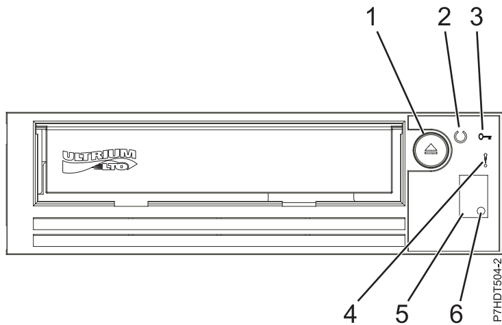
Figure 1. >Vue avant de l'unité LTO demi-hauteur
