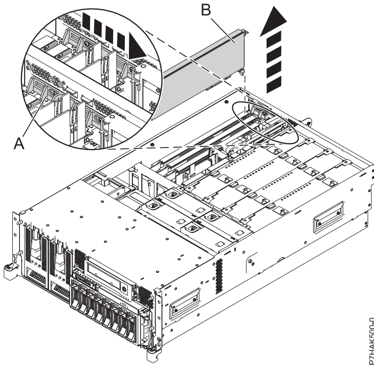
Figure 16. Retrait du panneau obturateur ou de la carte PCI d'une unité centrale montée en armoire
