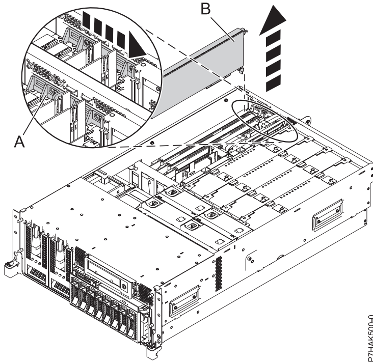
Figure 30. Retrait du panneau obturateur ou de la carte PCI d'une unité centrale montée en armoire
