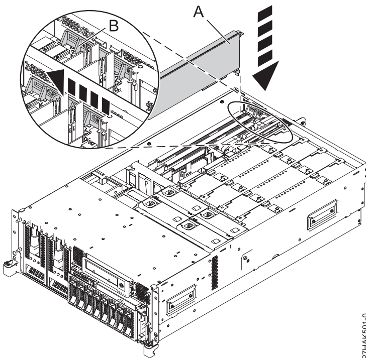
Figure 10. Remplacement de la carte PCI d'une unité centrale montée en armoire
