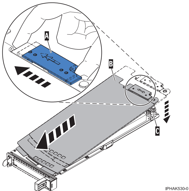
Figure 72. Réinstallation du couvercle de la cassette de cartes PCI
