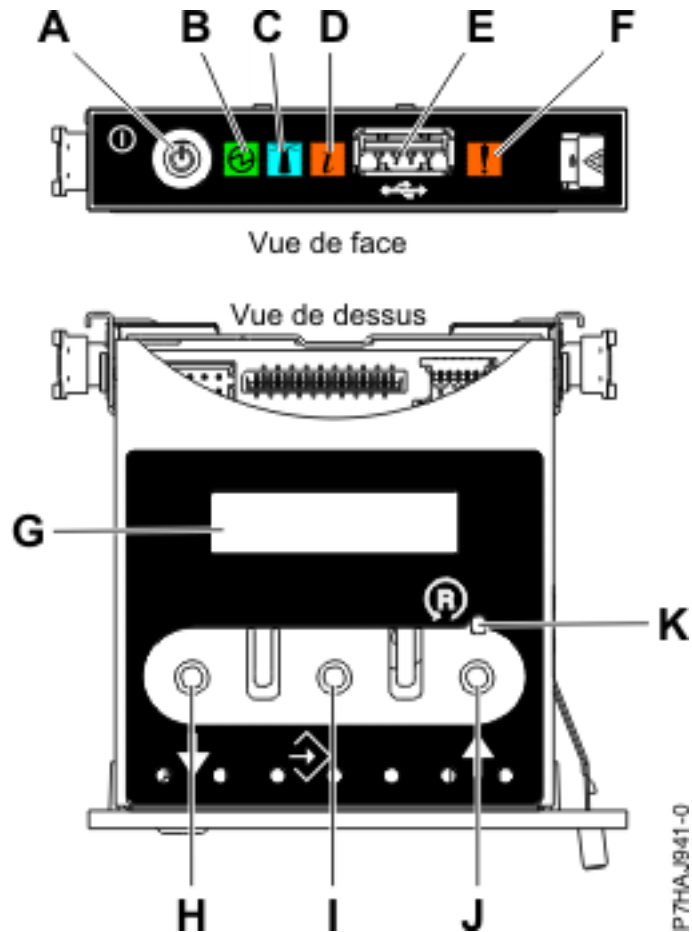
Figure 110. Panneau de commande
