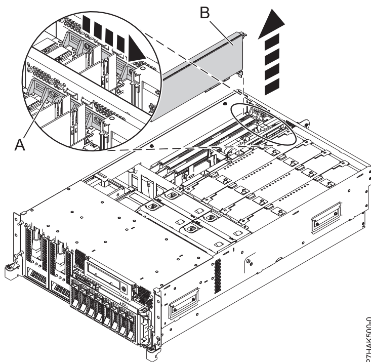
Figure 27. Retrait du panneau obturateur ou de la carte PCI d'une unité centrale montée en armoire
