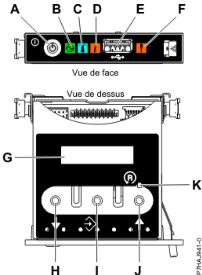
Figure 109. Panneau de commande
