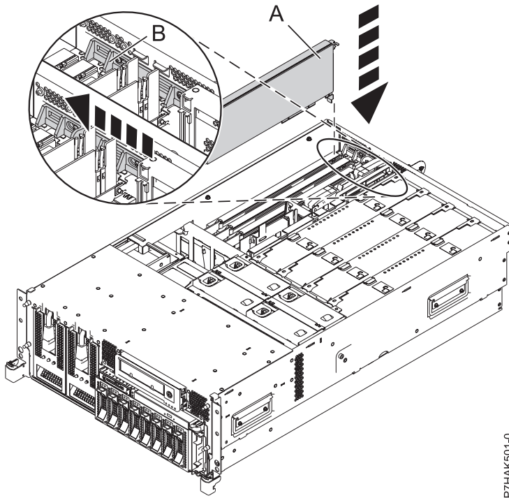
Figure 29. Remplacement de la carte PCI d'une unité centrale montée en armoire
