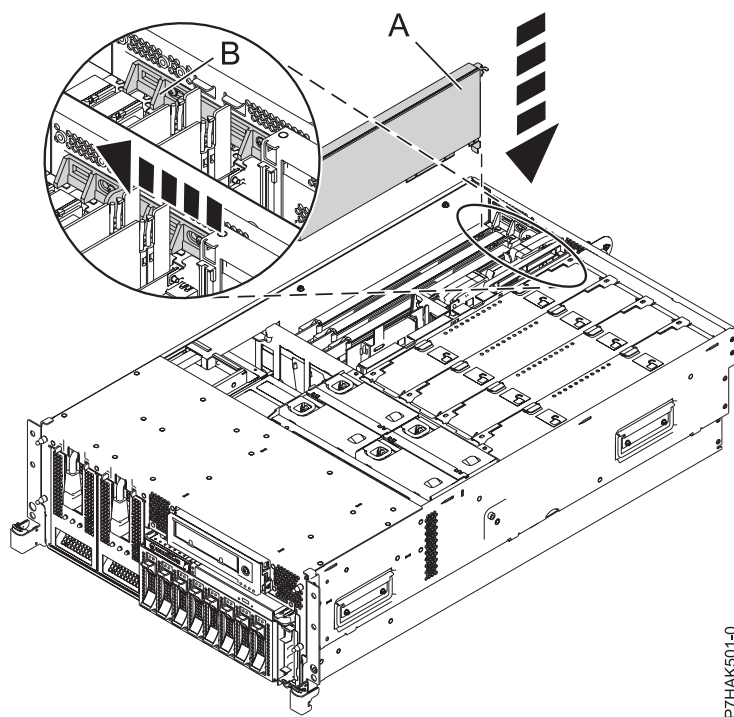
Figure 2. Remplacement de la carte PCI d'une unité centrale montée en armoire
