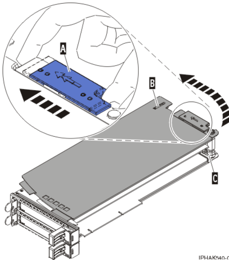
Figure 102. Réinstallation du couvercle de la cassette de cartes PCI
