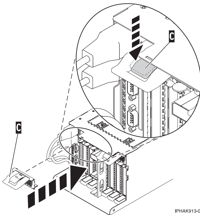
Figure 60. Blindage électromagnétique de la carte PCI en position fermée
