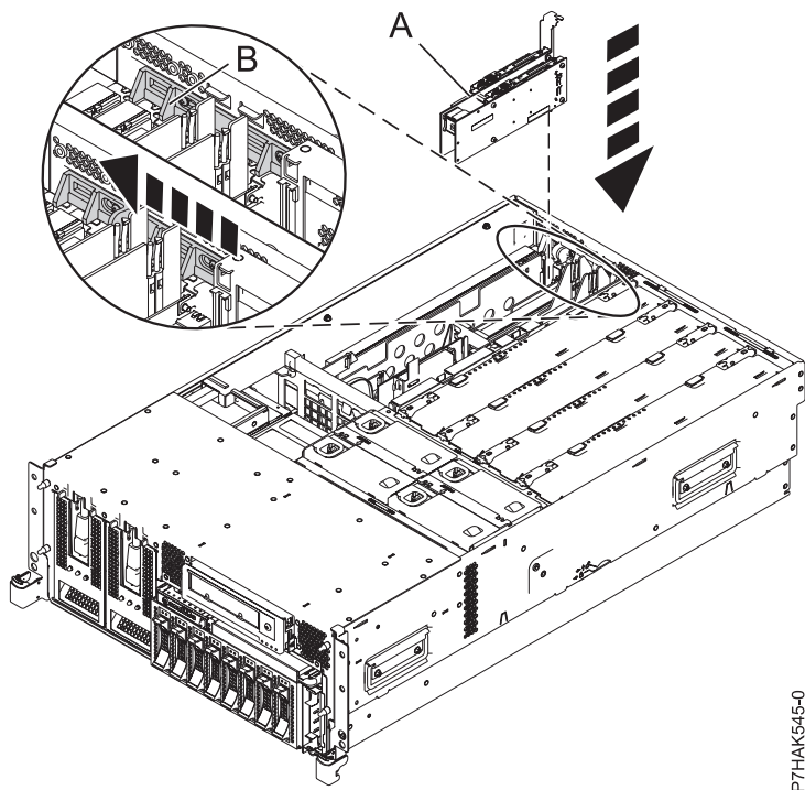
Figure 15. Remplacement de la carte PCIe RAID et SSD SAS d'une unité centrale montée en armoire
