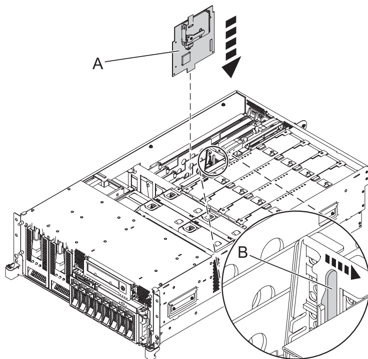
Figure 4. Modèle monté en armoire : remplacement de la carte de cache auxiliaire RAID
