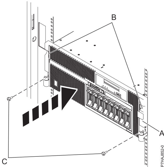
Figure 14. Installation du capot avant
