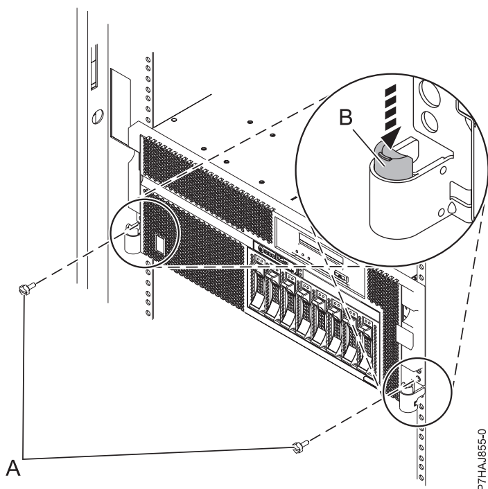
Figure 17. Déblocage des taquets de sécurité
