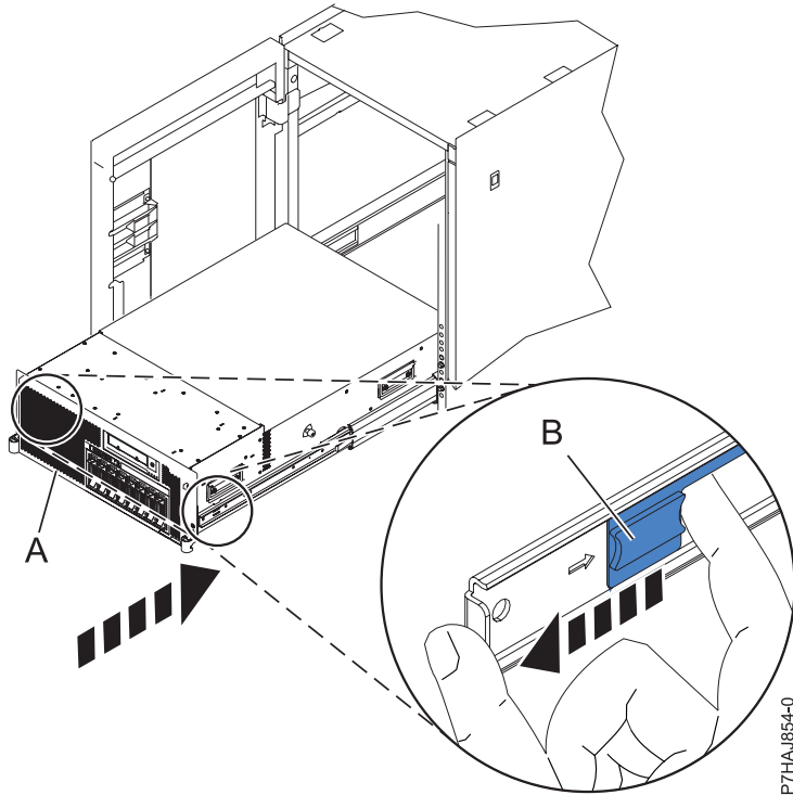
Figure 18. Déblocage des taquets de sécurité de la glissière
