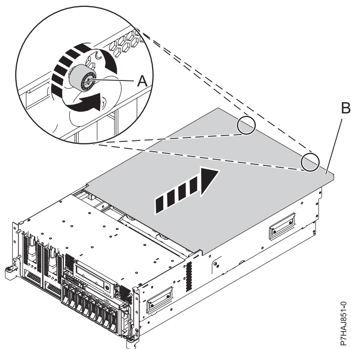
Figure 21. Retrait du capot d'accès
