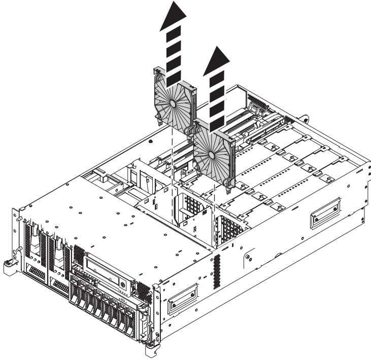
Figure 9. Retrait des grilles d'aération
