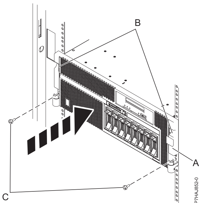
Figure 25. Remise en place des vis moletées
