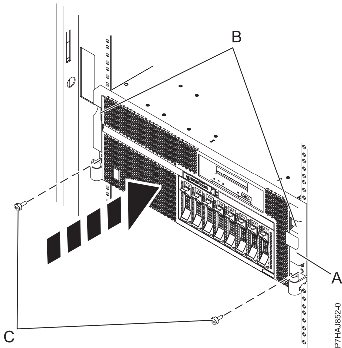
Figure 20. Installation du capot avant
