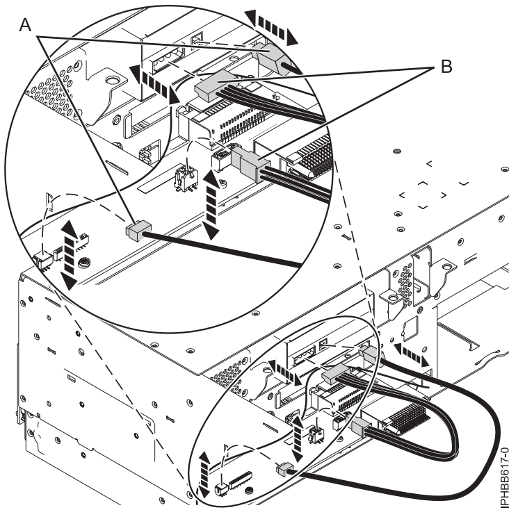
Figure 16. Fixation de l'unité de stockage (média) au fond de panier d'un système 33E/8B ou 36E/8C
