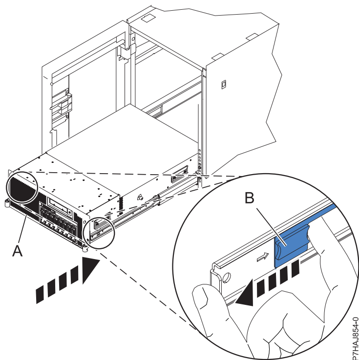
Figure 24. Déblocage des taquets de sécurité de la glissière
