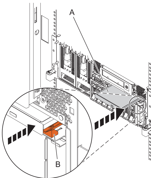
Figure 7. Installation d'une unité de stockage (média) extra-plate
