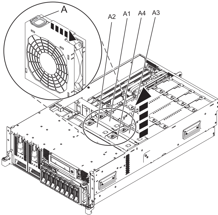
Figure 4. Retrait du ventilateur
