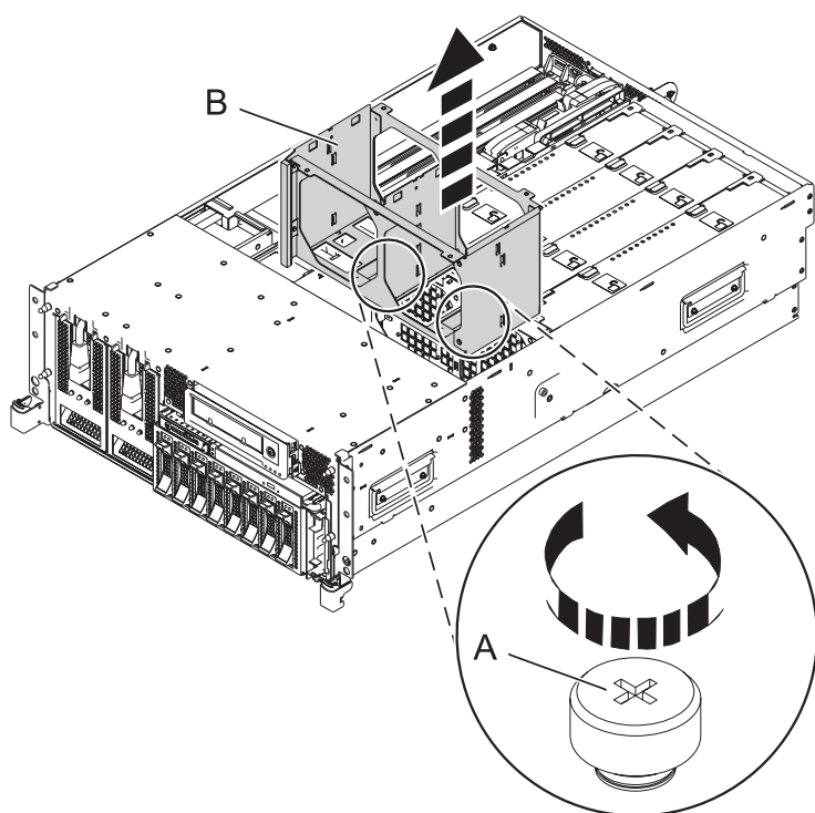
Figure 3. Retrait du boîtier de ventilation
