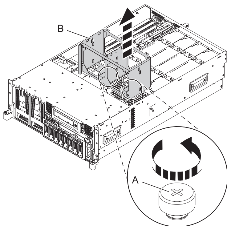
Figure 12. Retrait du boîtier de ventilation
