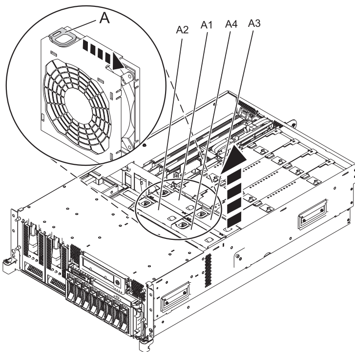
Figure 8. Retrait du ventilateur
