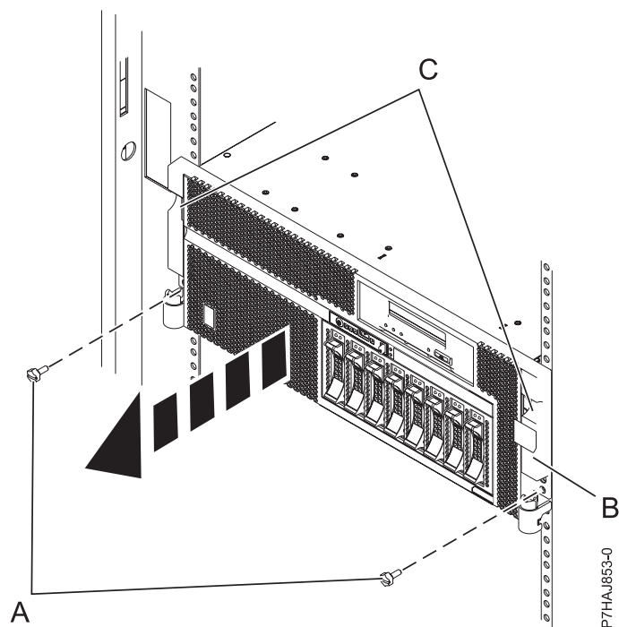
Figure 19. Retrait du capot avant
