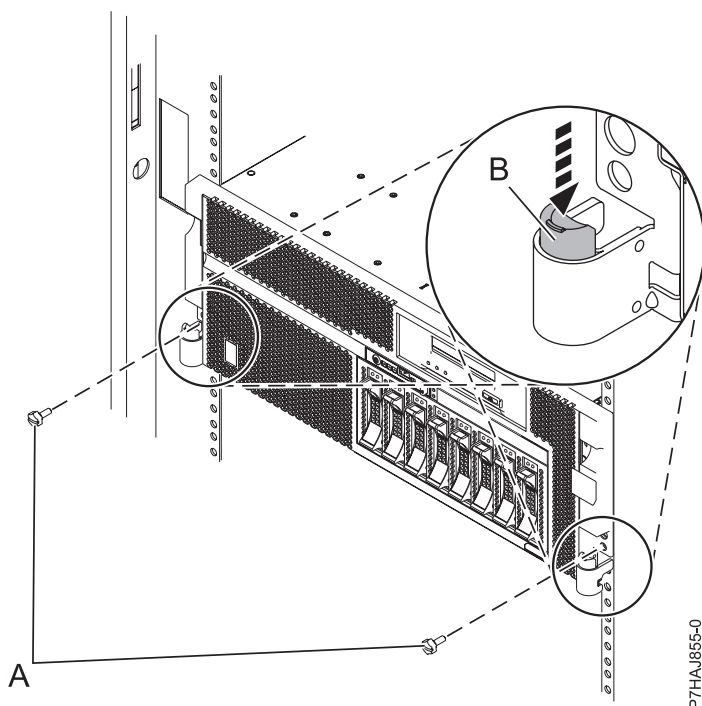
Figure 23. Déblocage des taquets de verrouillage
