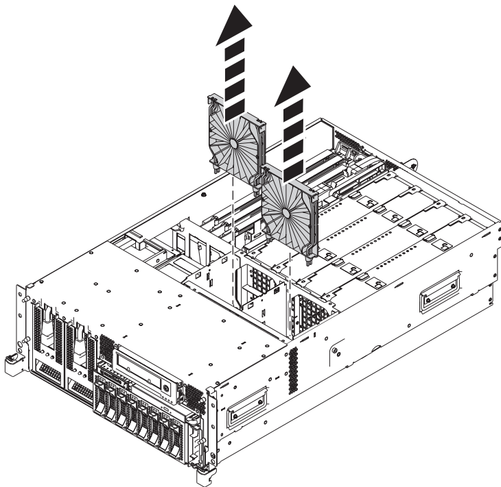
Figure 5. Retrait des grilles d'aération
