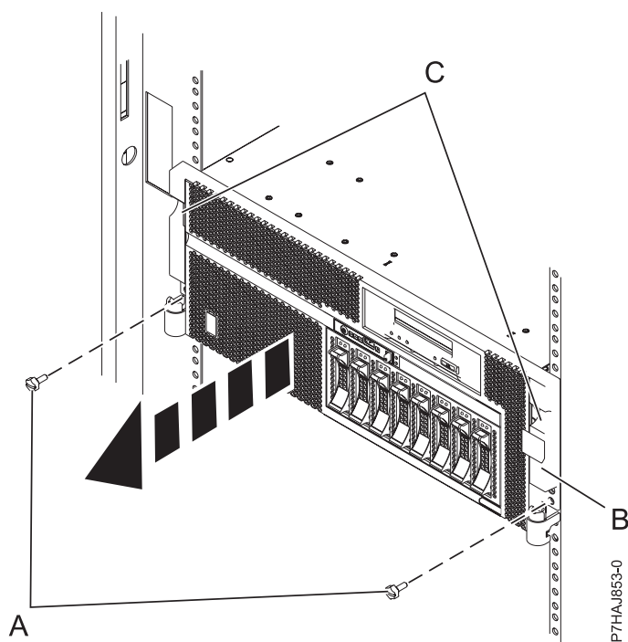
Figure 4. Retrait du capot avant
