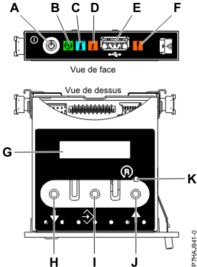
Figure 1. Panneau de commande
