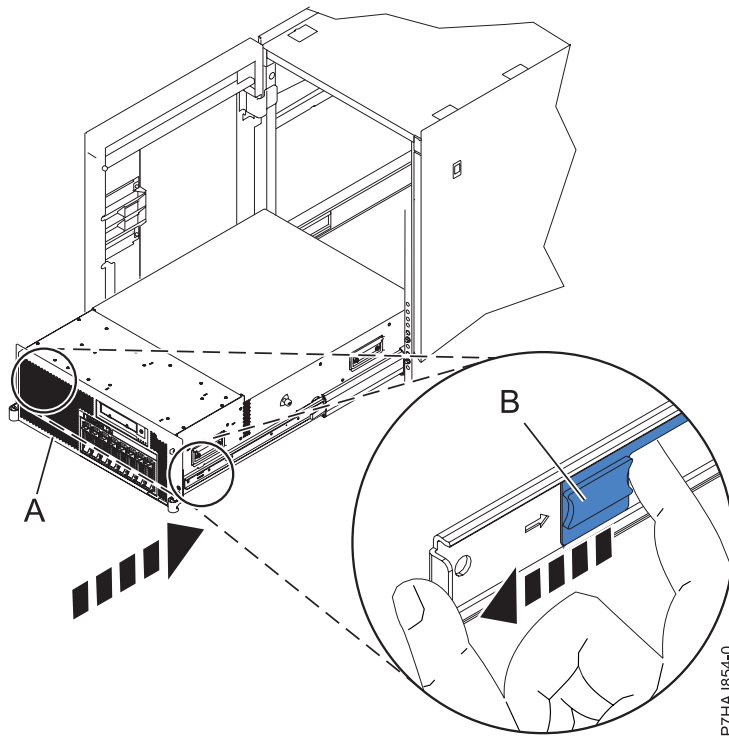
Figure 7. Déblocage des taquets de sécurité de la glissière
