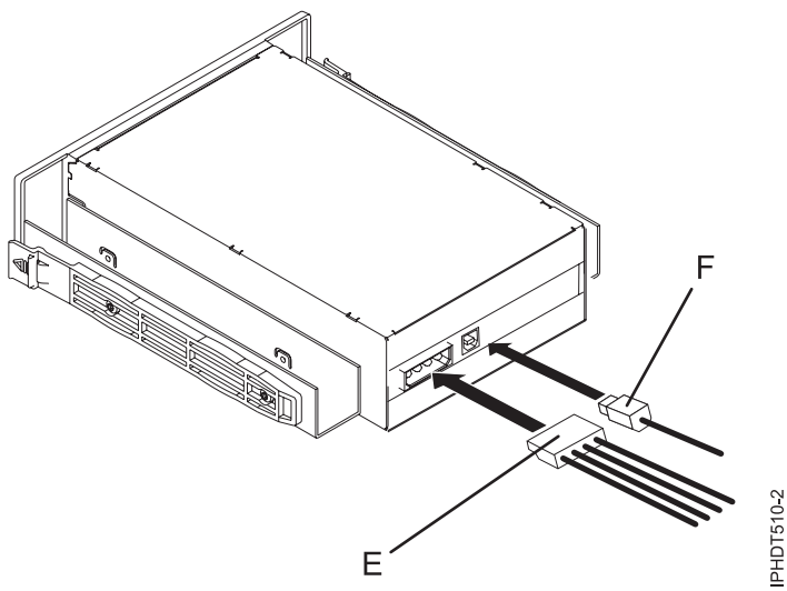
Figure 14. Unité interne, vue arrière et connecteurs
