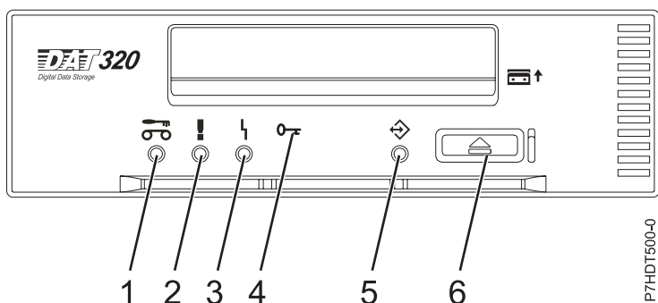
Figure 11. Vue avant de l'unité de bande
