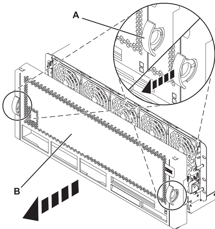
Figure 79. Retrait du capot avant
