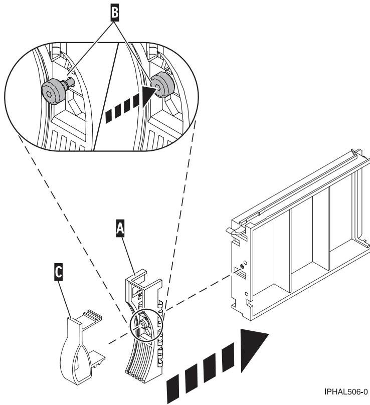
Figure 30. Fixation d'un panneau frontal à un obturateur d'unité de disque
