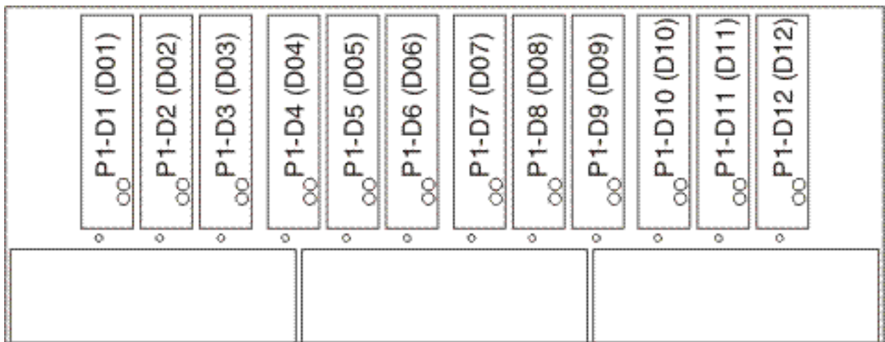
Figure 45. Vue de face des boîtiers d'unités de disque SCSI 31D/24 et 31T/24
