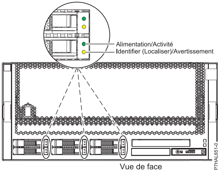
Figure 39. Emplacements des voyants d'activité des unités de disque sur le système
