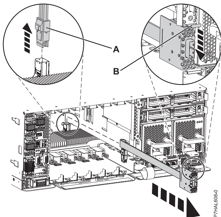
Figure 34. Retrait du câble SAS
