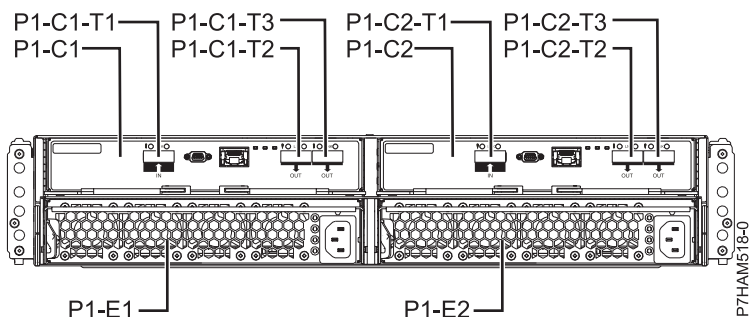
Figure 41. Vue arrière du Boîtier d'unité de disque 58/87
