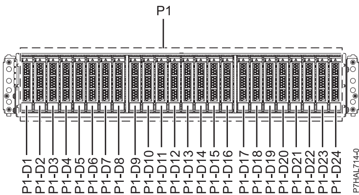
Figure 40. Vue de face du Boîtier d'unité de disque 58/87 illustrant les emplacements des unités de disque
