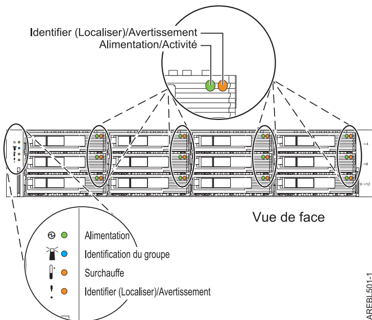
Figure 44. Vue de face des voyants d'activité sur le boîtier d'unité de disque 58/86
