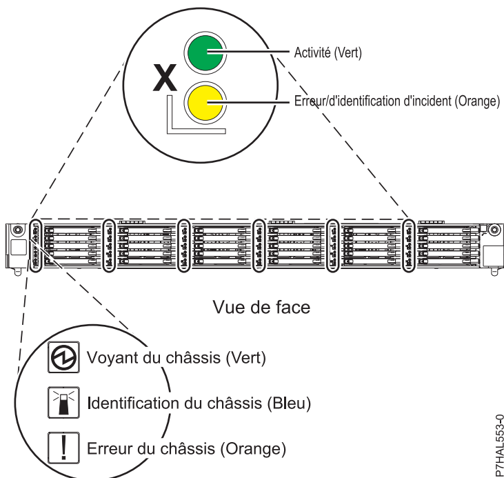
Figure 51. Vue de face de l'armoire de stockage PCIe ED/R1 illustrant les voyants d'activité
