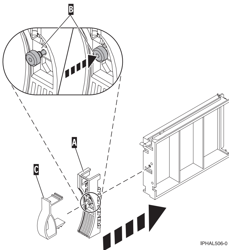
Figure 33. Fixation d'un panneau frontal à un obturateur d'unité de disque
