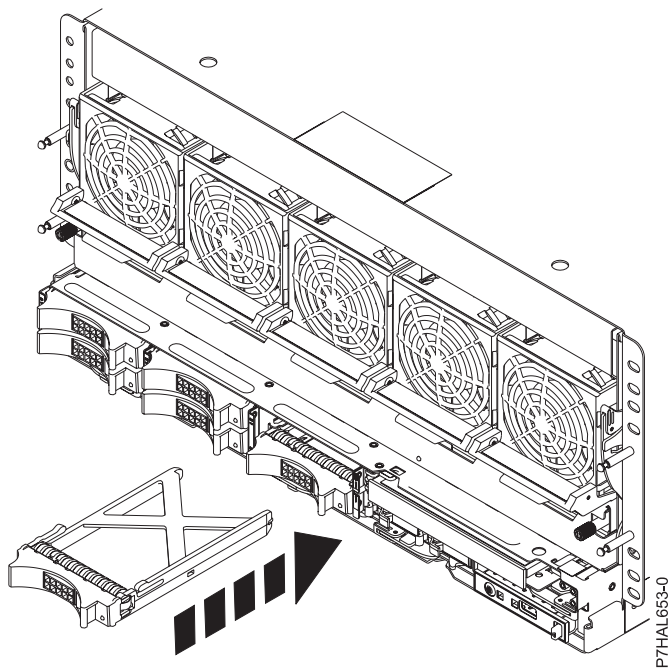
Figure 31. Installation d'un obturateur d'unité de disque
