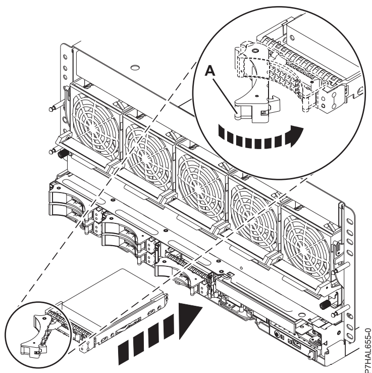
Figure 25. Remplacement d'une unité de disque dans l'unité centrale
