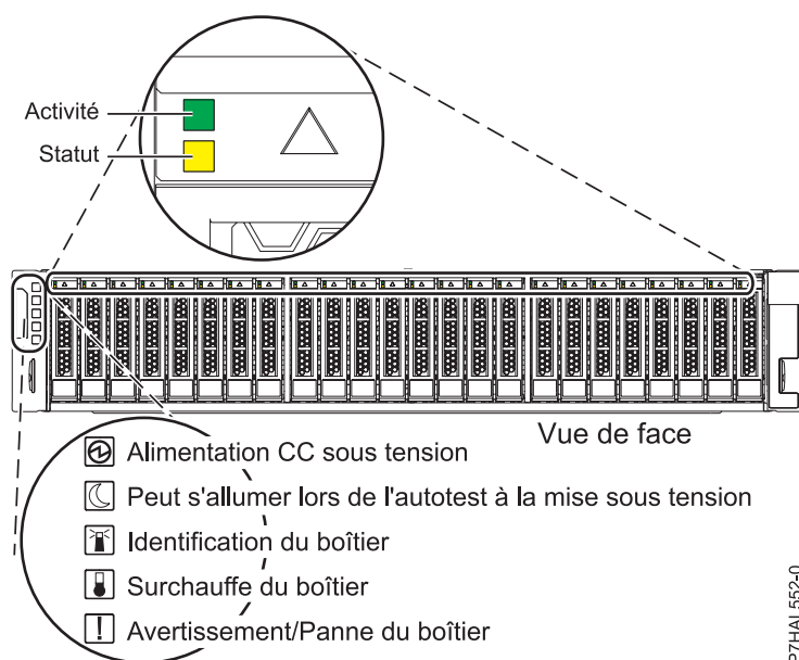
Figure 42. Vue de face du Boîtier d'unité de disque 58/87 illustrant les voyants d'activité
