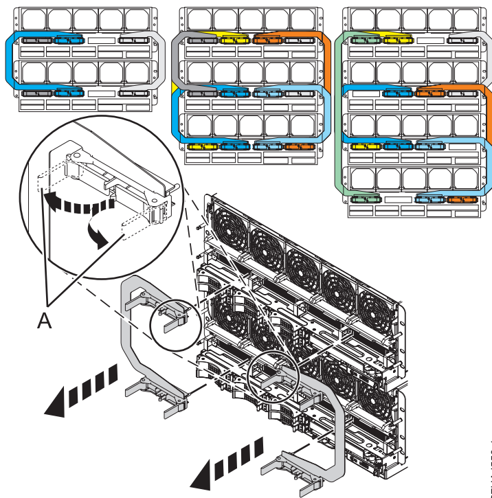
Figure 11. Déconnexion du câble SMP
