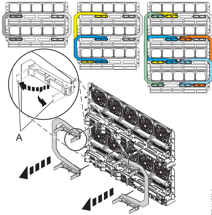
Figure 10. Déconnexion du câble SMP
