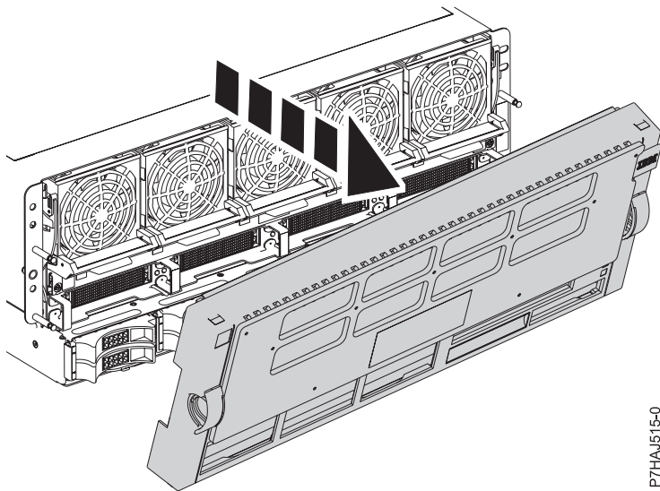
Figure 21. Retrait du capot
