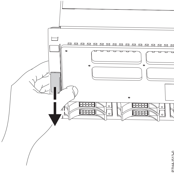
Figure 19. Déblocage des taquets de sécurité du capot
