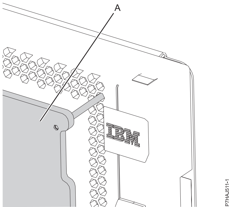
Figure 17. Alignement de l'outil de retrait de capot
