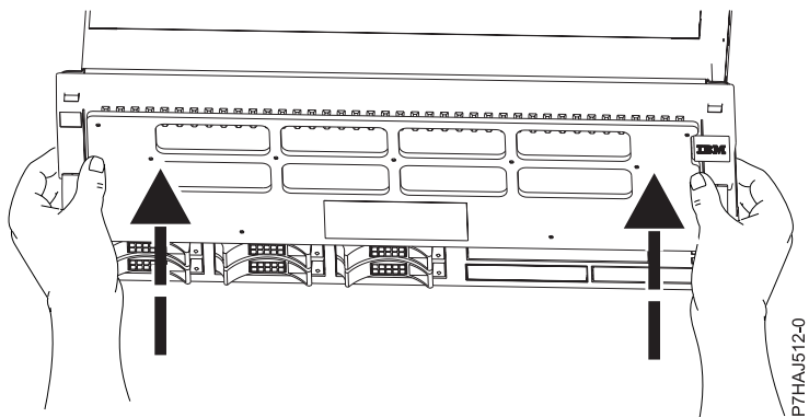
Figure 18. Utilisation de l'outil de retrait de capot
