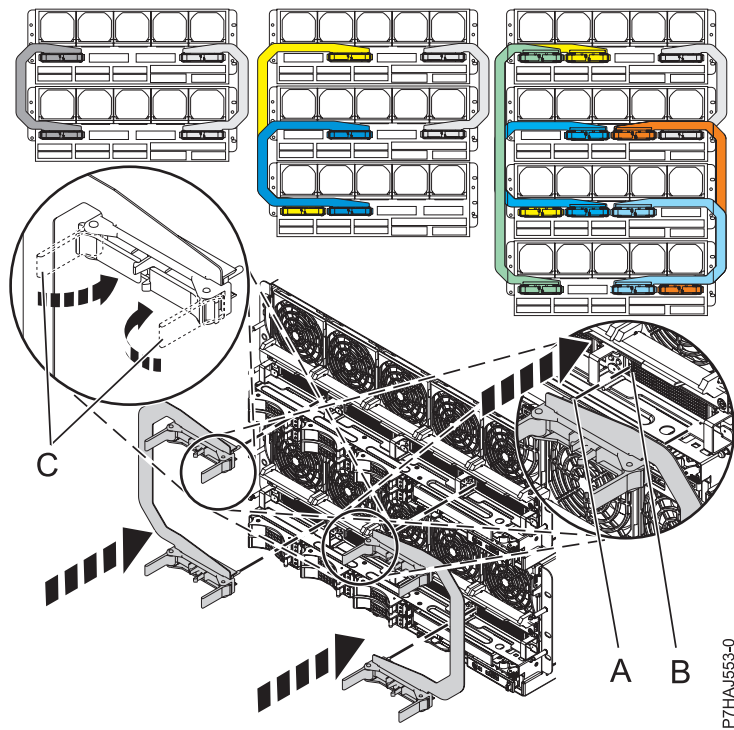
Figure 12. Reconnexion du câble SMP
