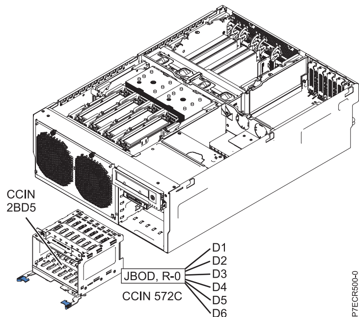
Figure 4. Baies de disques contrôlées par le fond de panier de base
