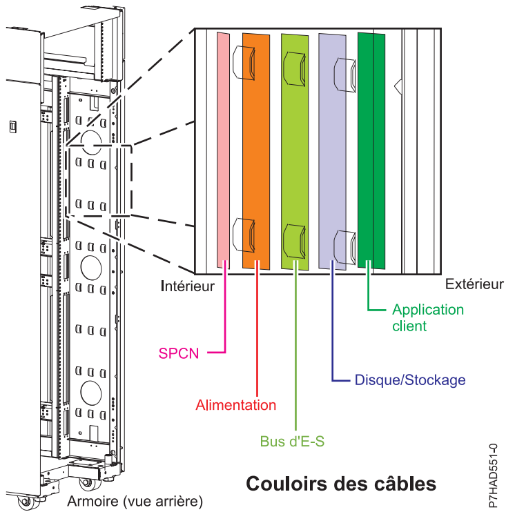
Figure 13. Ponts lance de gestion des câbles
