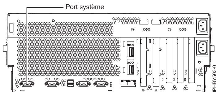
Figure 9. Connexion pour les modèles 8233-E8B et 8236-E8C
