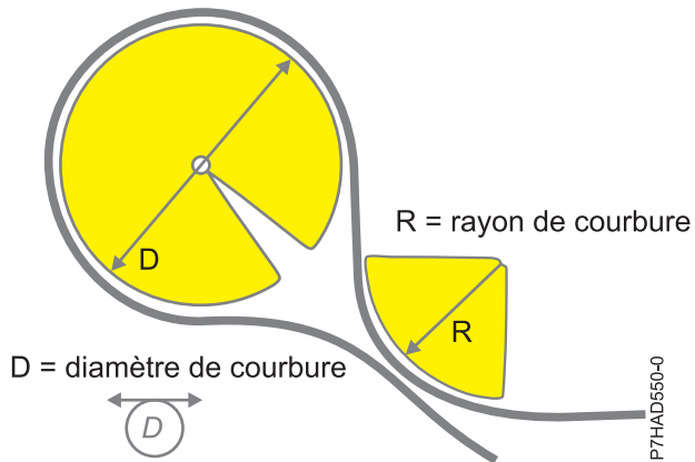
Figure 14. Rayon de courbure du câble
