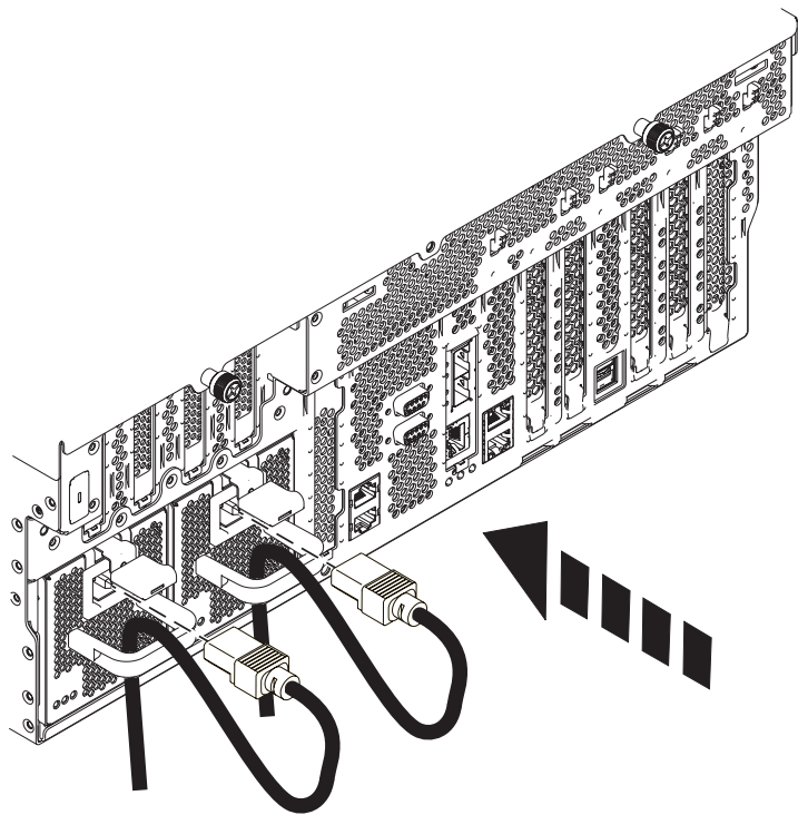
Figure 12. Fixation et routage du cordon d'alimentation
