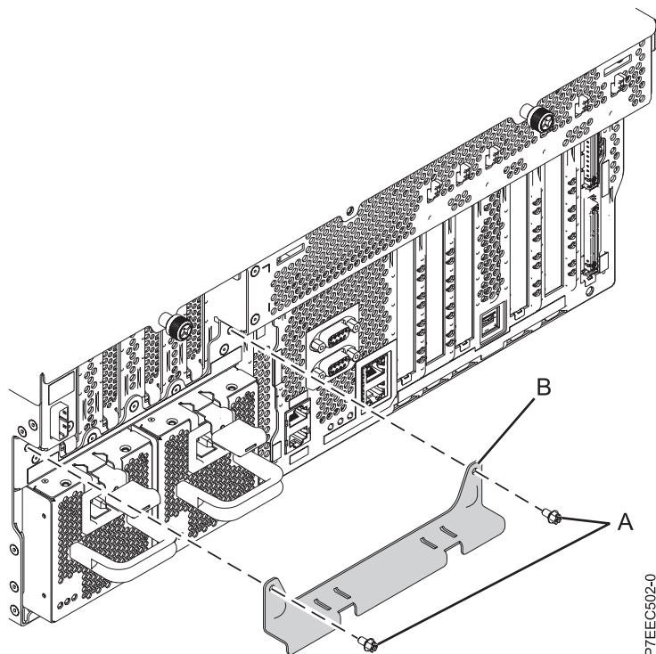
Figure 11. Retrait du support de transport
