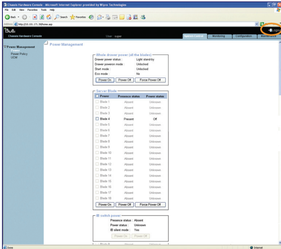
Figure 2-4. Déconnexion de la console CHC (Chassis Hardware Console)
