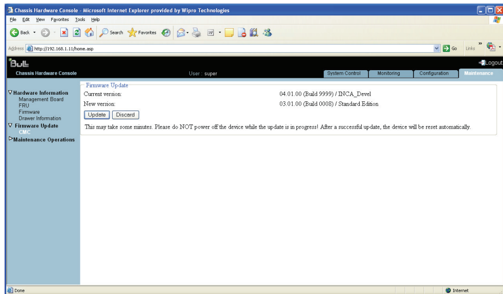
Figure 6-6. Page Firmware Upload - Step2 (Téléchargement du micrologiciel - Etape 2)
