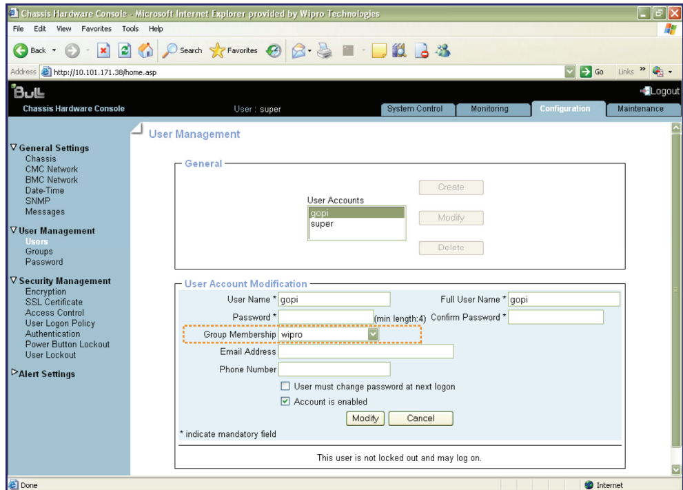
Figure 5-25. Boîte User Account Modification (Modification de compte utilisateur)
