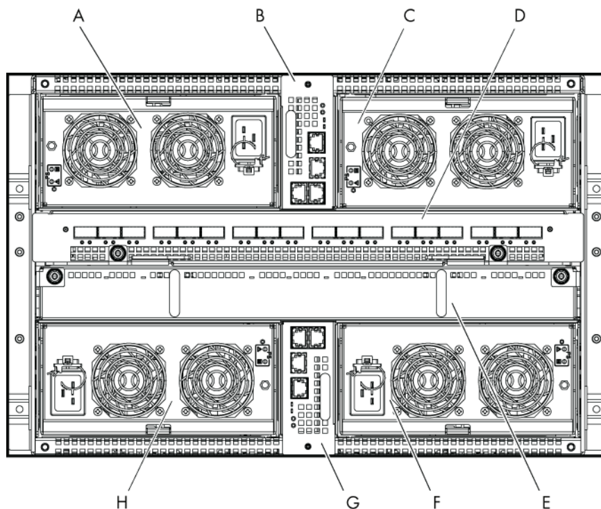
Figure 1-8. Vue arrière
