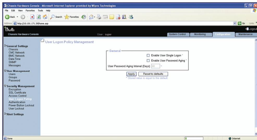
Figure 5-29. Page User Logon Policy Management (Gestion des politiques d'ouverture de session des utilisateurs)
