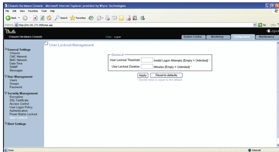
Figure 5-32. Page User Lockout Management (Gestion des verrouillages utilisateur)
