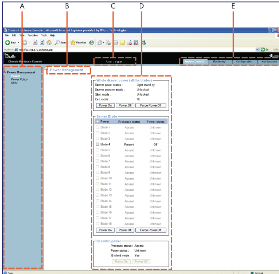
Figure 2-3. Présentation générale de la console CHC (Chassis Hardware Console)
