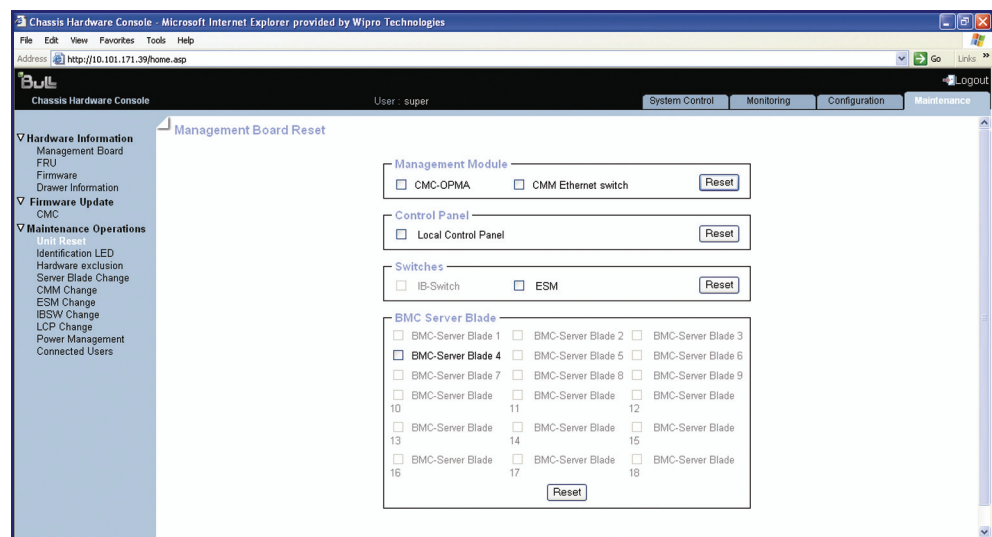
Figure 6-8. Page Management Board Reset (Réinitialisation de la carte de gestion)
