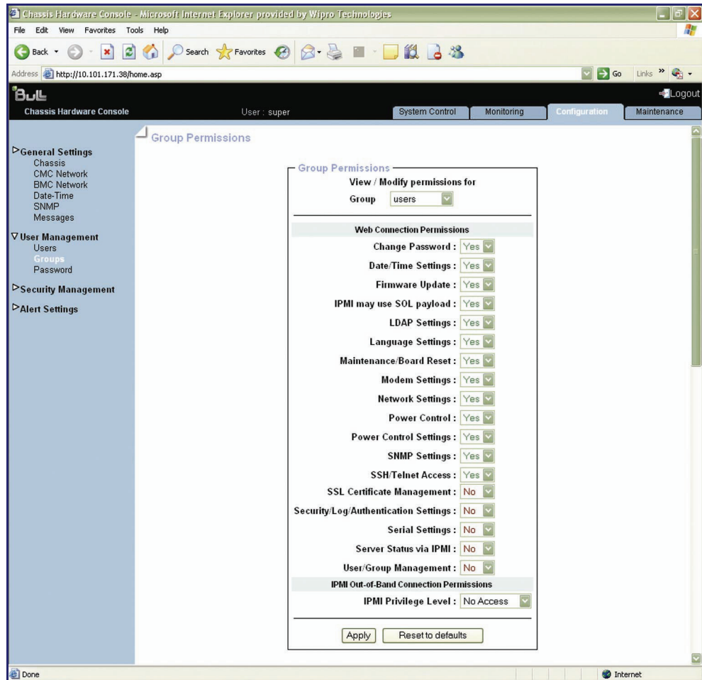
Figure 5-23. Page Group Permissions (Autorisations de groupe)
