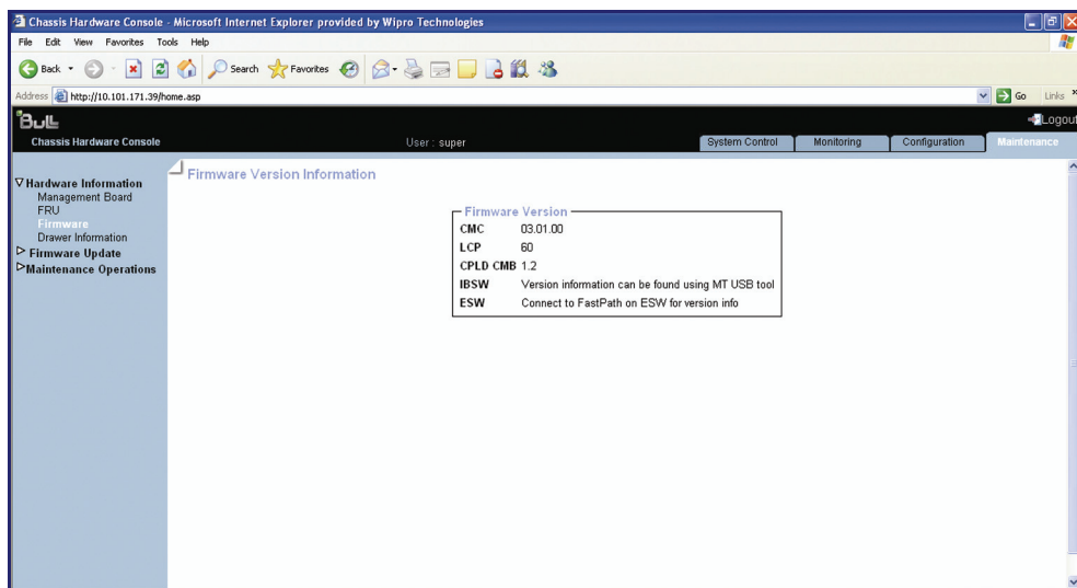
Figure 6-3. Page Firmware Version Information (Informations sur la version du micrologiciel)
