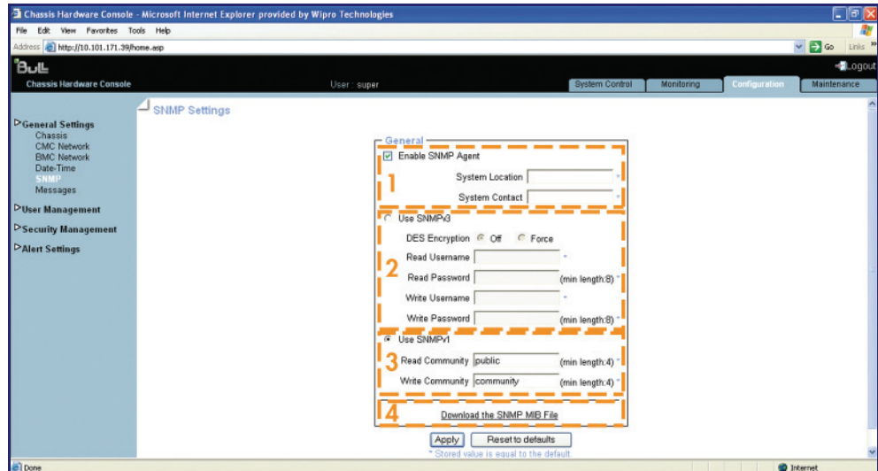
Figure 5-5. Page SNMP Settings (Paramètres SNMP)
