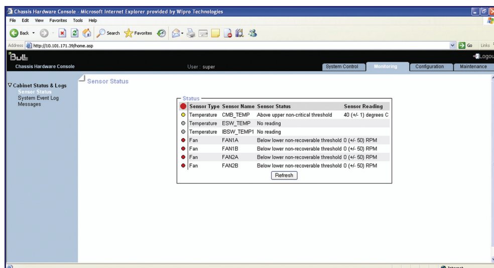
Figure 4-1. Page Sensor Status (Etat des capteurs)
