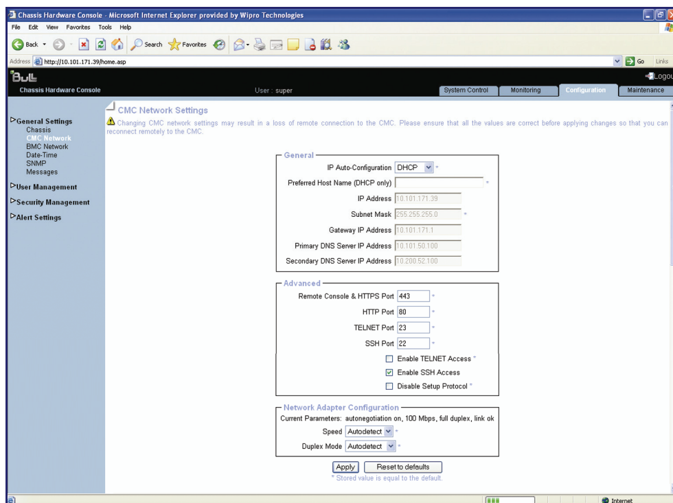
Figure 5-2. Page CMC Network Setting (Paramètre réseau du CMC)
