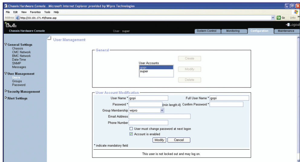
Figure 5-10. Boîte User Account Modification (Modification de compte utilisateur)
