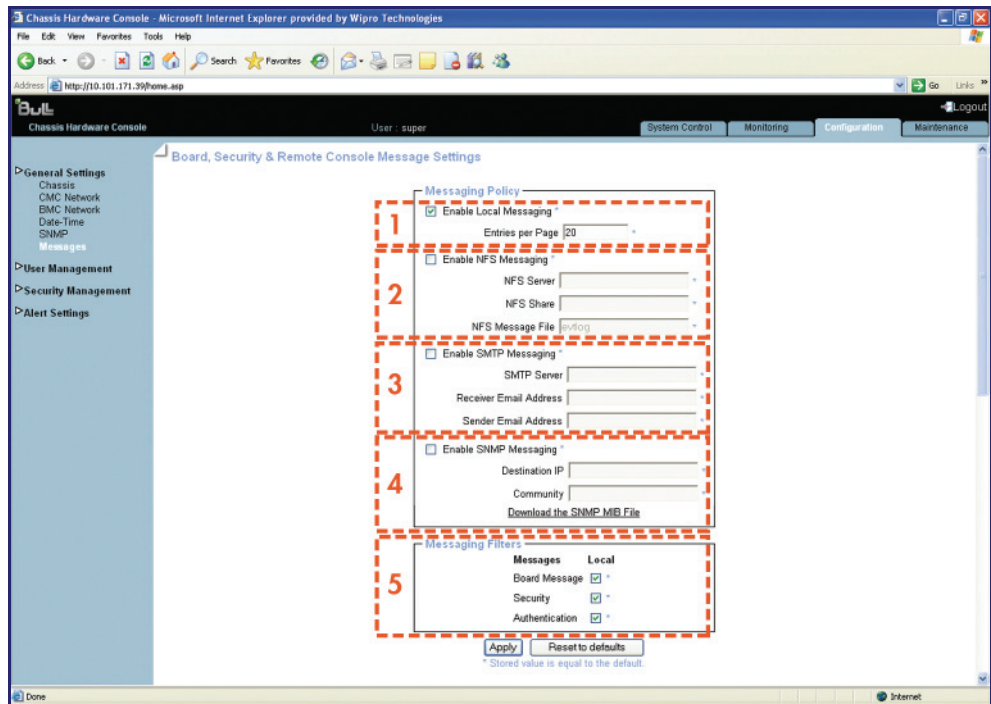
Figure 5-6. Page Board, Security & Remote Console Messages Settings (Paramètres des messages console distante, sécurité et cartes)
