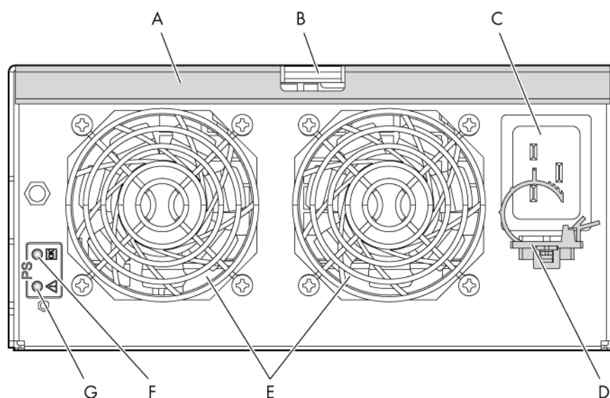
Figure 1-9. Module d'alimentation
