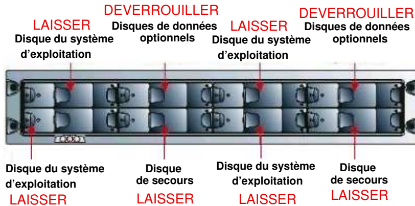
Figure 48. Sous-systèmes disques SJ-0812 SCSI JBOD – Tous domaines
