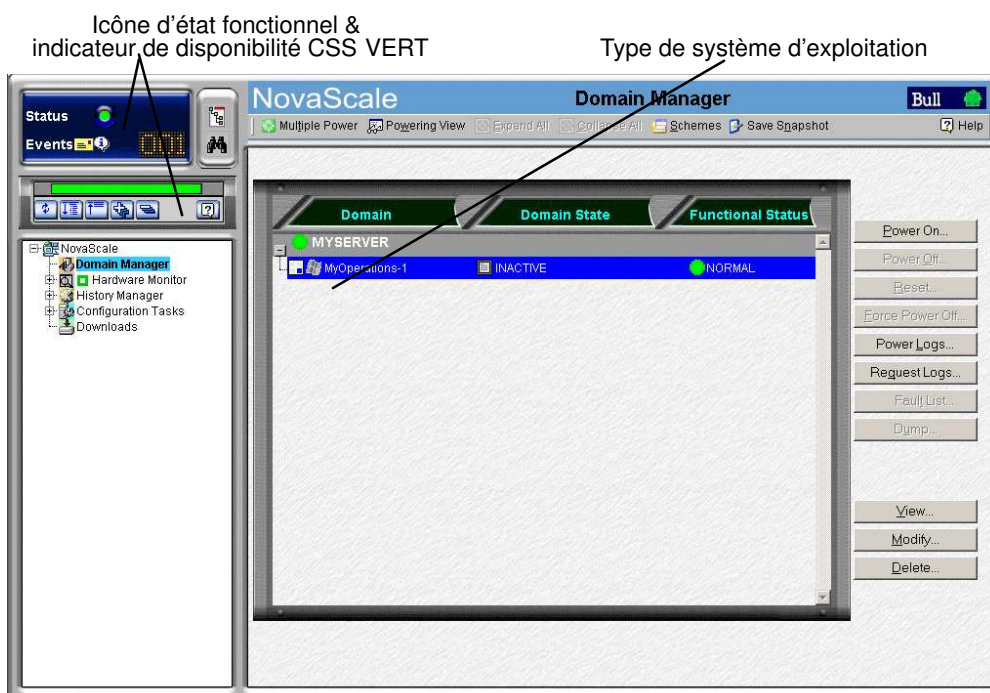
Figure 32. Volet de commandes du gestionnaire de domaines
