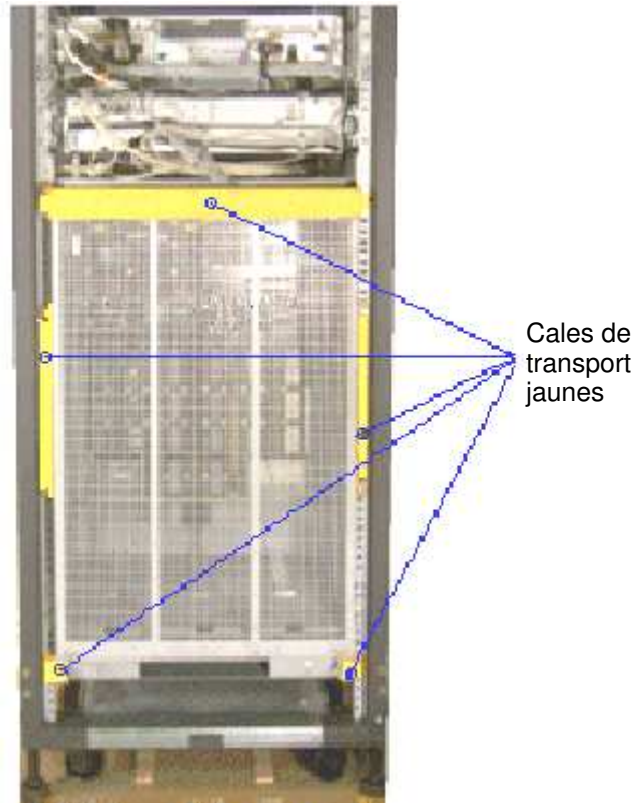
Figure 2. Retrait des cales de transport du module CSS – Arrière de l'armoire 36U
