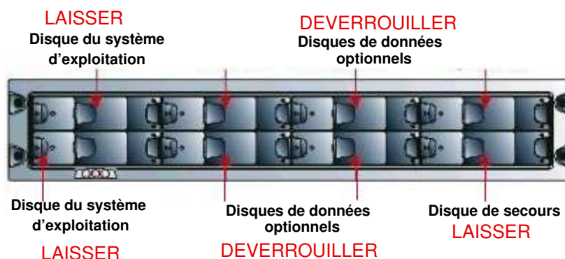
Figure 49. Sous-systèmes disques SR-0812 SCSI RAID – Tous domaines
