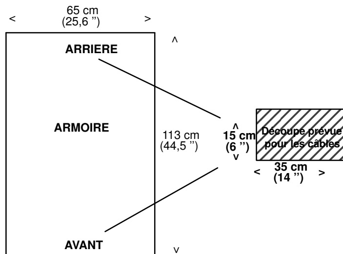
Figure 27. Découpes prévues pour les câbles de l'armoire
