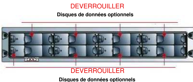
Figure 50. Position des disques d'extension SJ-0812 (données) – Tous domaines
