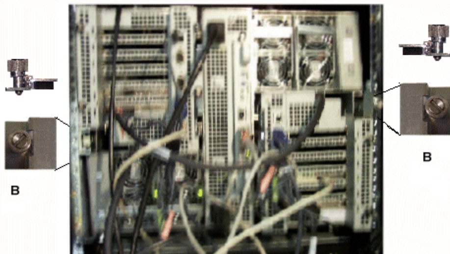
Figure 5. Installation des butées arrière
