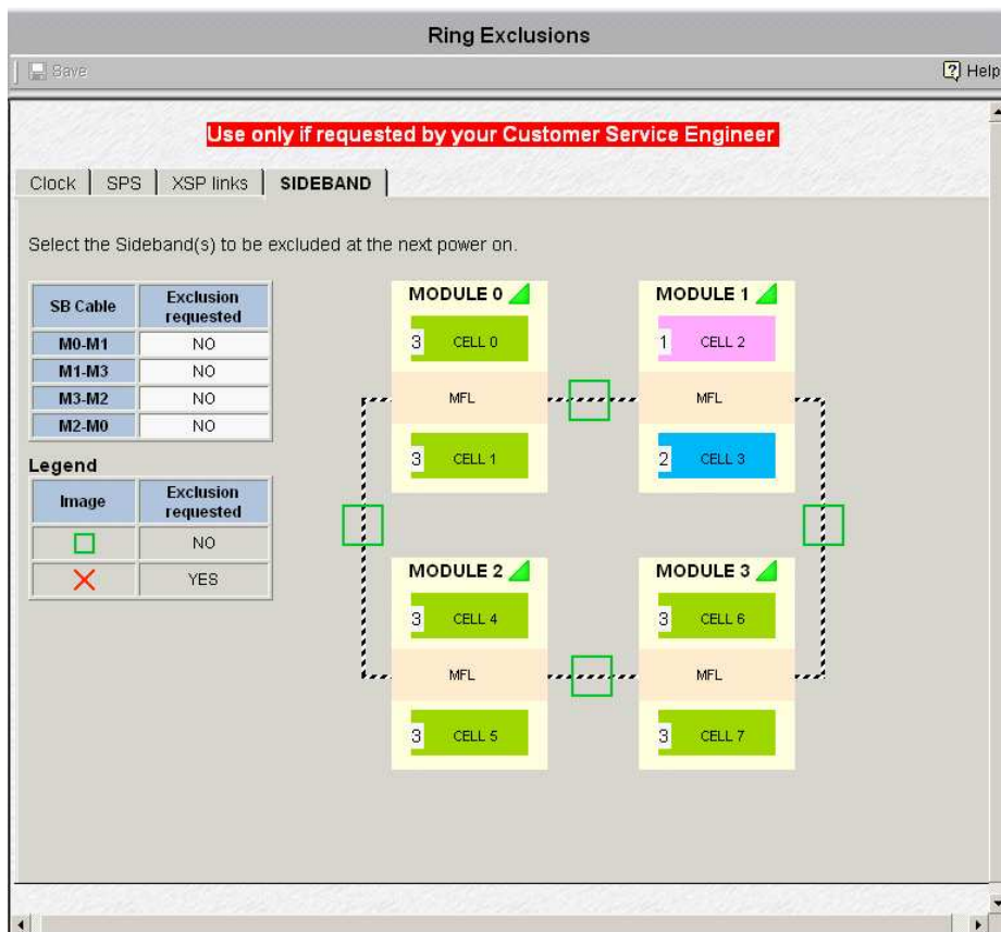
Figure 83. Volet de commandes de Ring exclusion (Exclusion de l'anneau) - onglet Sideband (Bande latérale)
