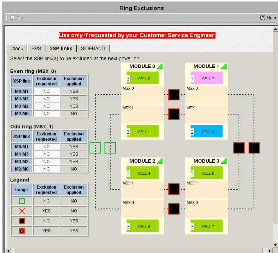
Figure 82. Volet de commandes de Ring exclusion (Exclusion de l'anneau) - onglet XSP link (Liaison XSP)
