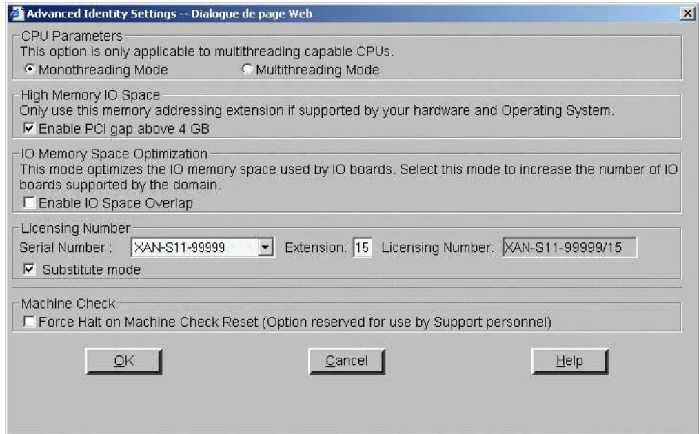
Figure 165. Boîte de dialogue Advanced Identity Settings (Paramètres d'identité avancés) - Exemple 4
